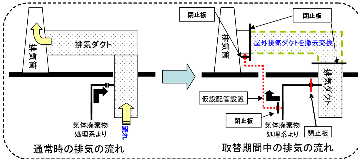
気体廃棄物処理系仮設配管設置工事(平成22年10月25日設置済み)
