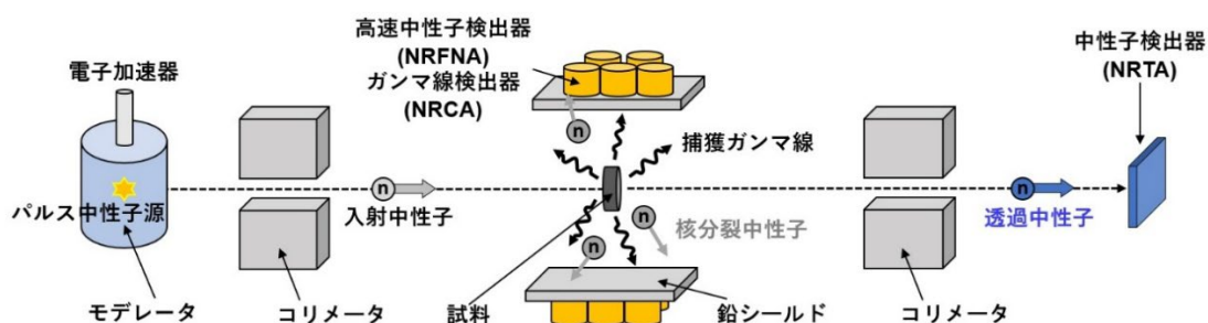
図1 NRA法の概念図
