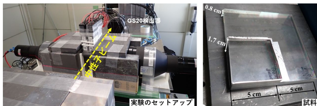
図 2 NRTA 実験の配置図と石英ガラス試料
