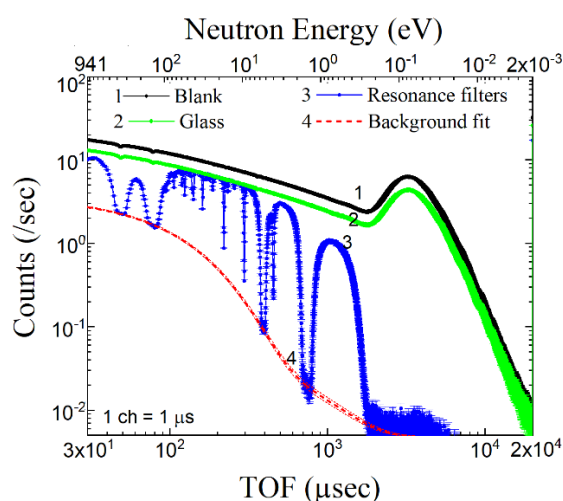
図 3 得られた TOF スペクトル [5]
