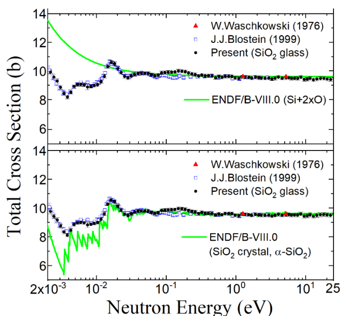
図 4 得られた石英ガラスの中性子全断面積 [5]
