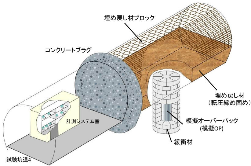
人工バリア性能確認試験の概要
