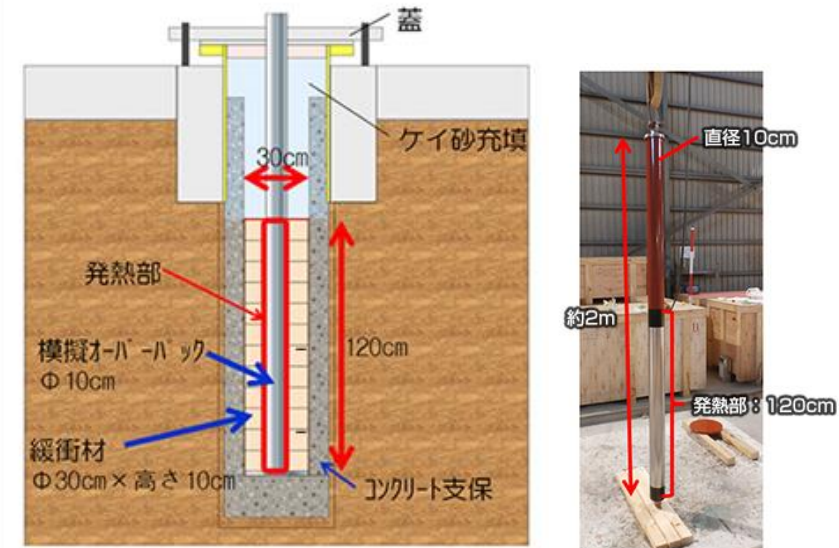
オーバーパック腐食試験の概念図
