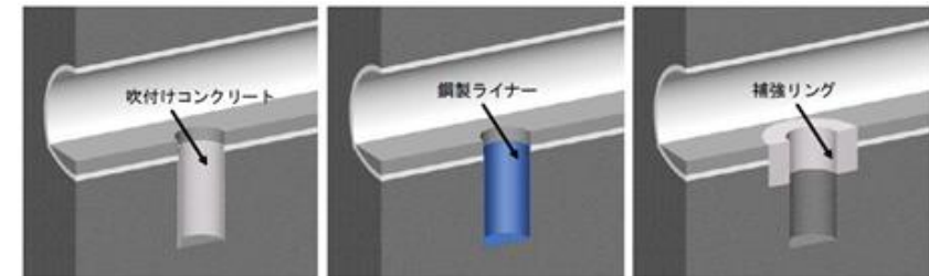
支保工設計と適用事例
