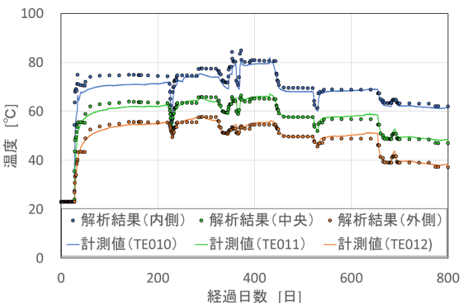
緩衝材中の温度
