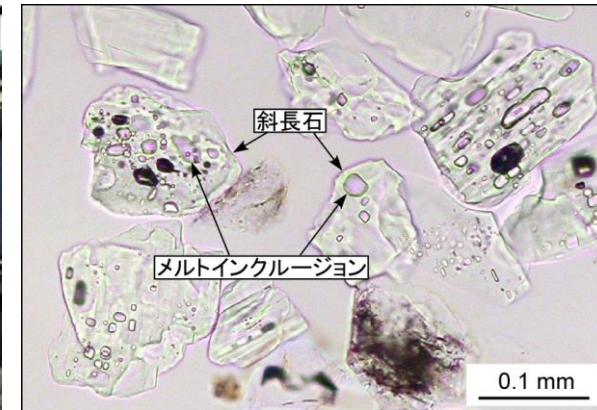
粘土質せん断帯に含まれるメルトインクルージョンの顕微鏡写真
