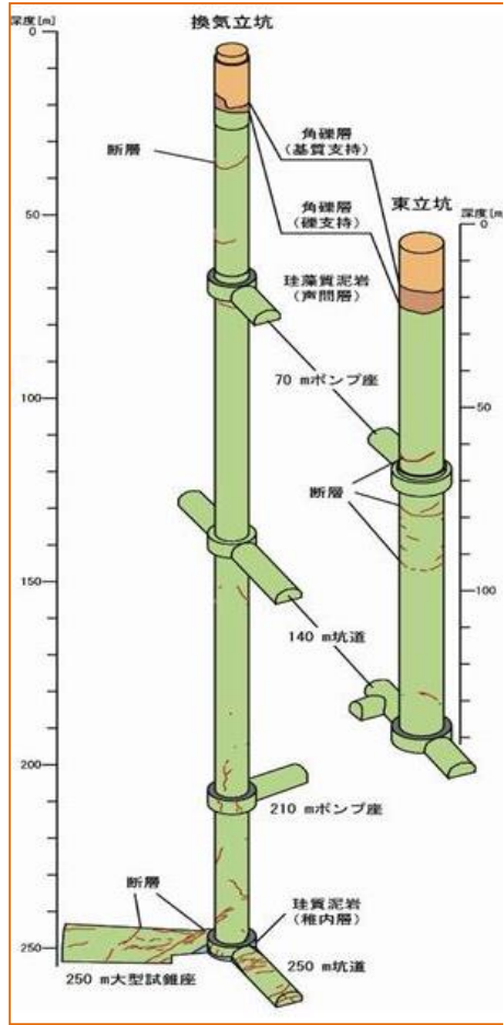
坑道壁面の地質観察
