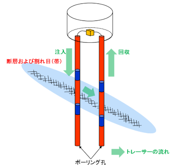
原位置トレーサー試験
