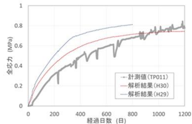
緩衝材中の土圧
