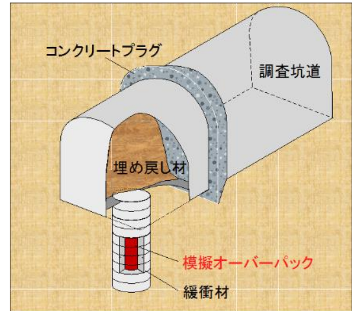
人工バリア性能確認試験の概要
