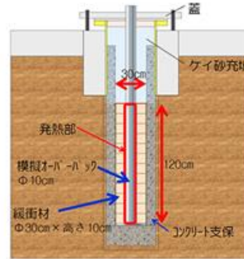
オーバーバック腐食試験
