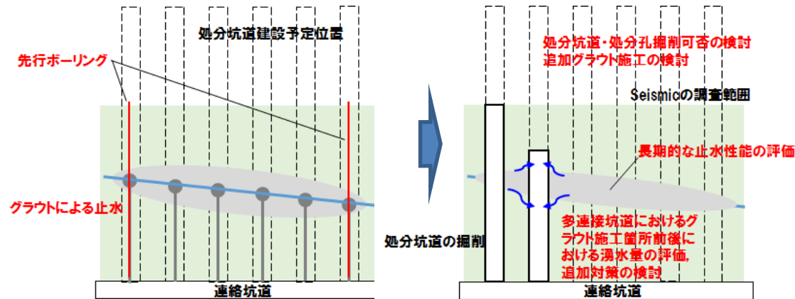
設計評価、工学的対策の検討イメージ
