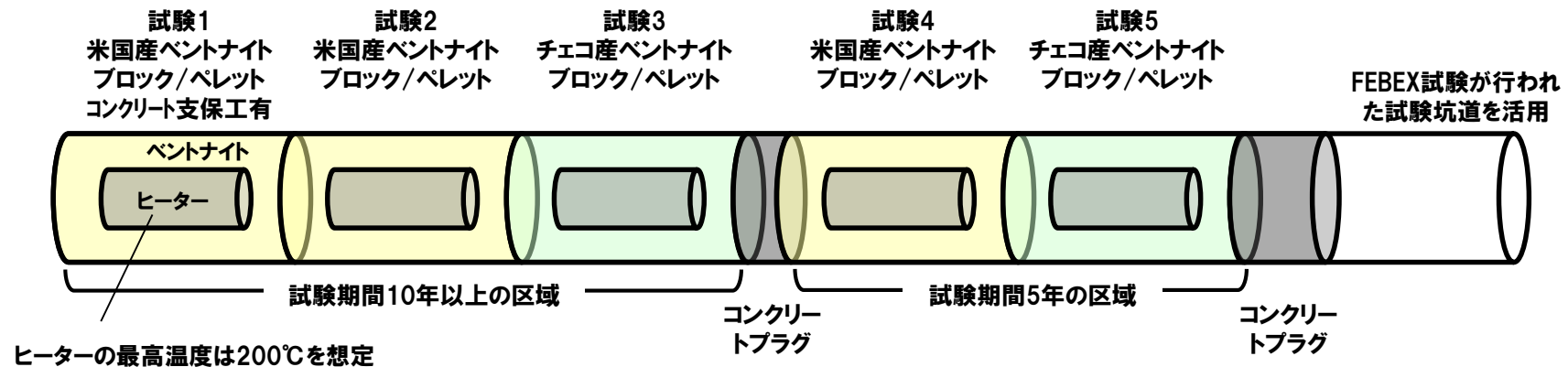
国際プロジェクトHotBENT試験の概要
