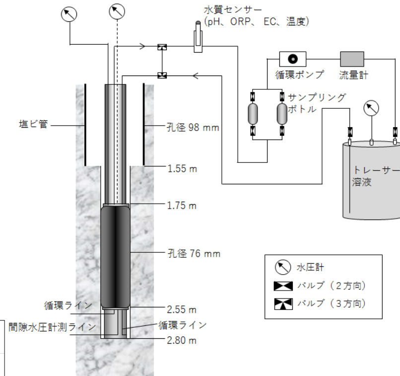
トレーサー試験装置の概念図
