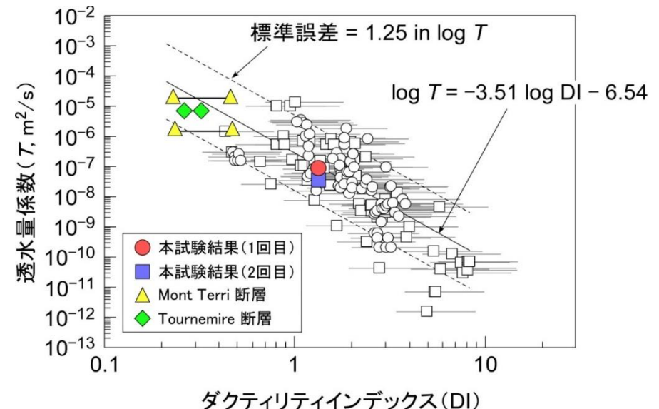
ダクティリティインデックスの経験式と今回実施した水圧擾乱試験結果や他の既報データとの比較
