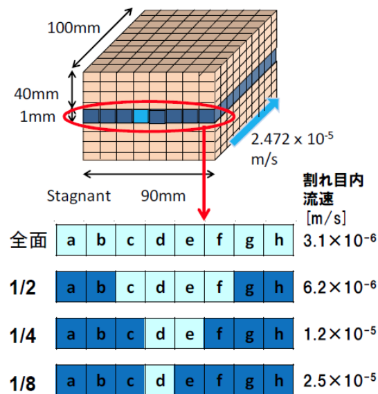
不均質な流れを仮定したモデル
