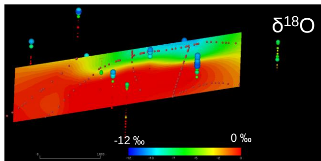
地下水の \text{Cl}^- 及び \delta^{18}\text{O} 分布の推定例
