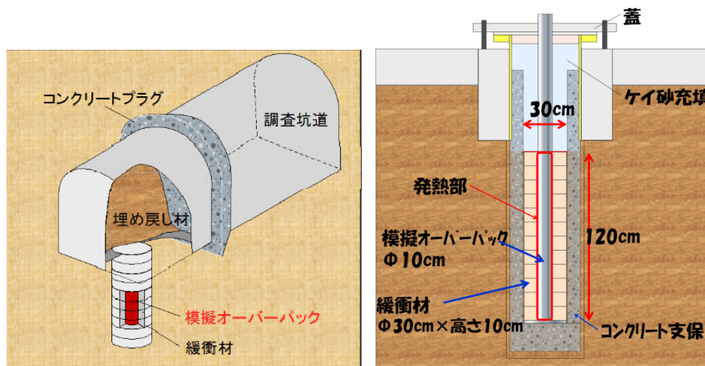
人工バリア性能確認試験
