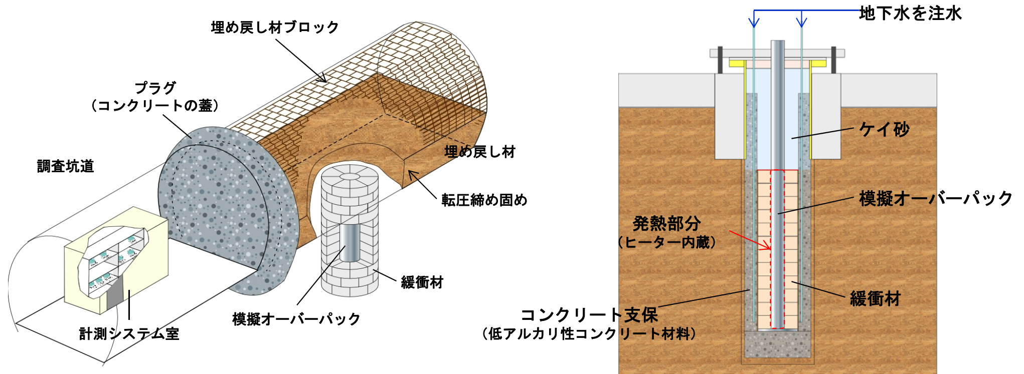
熱－水理－力学－化学連成挙動に関する試験 (人工バリア性能確認試験) の概念図
