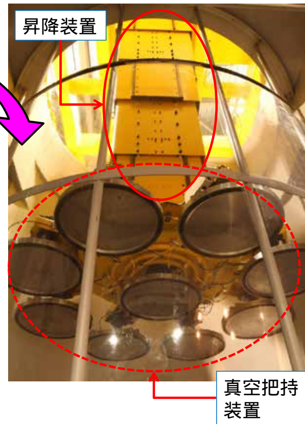
緩衝材の定置試験設備の製作状況
