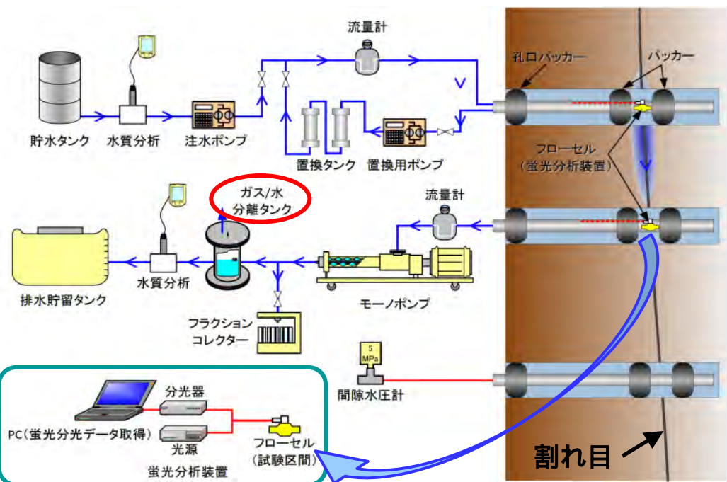
物質移行試験装置の概念図
