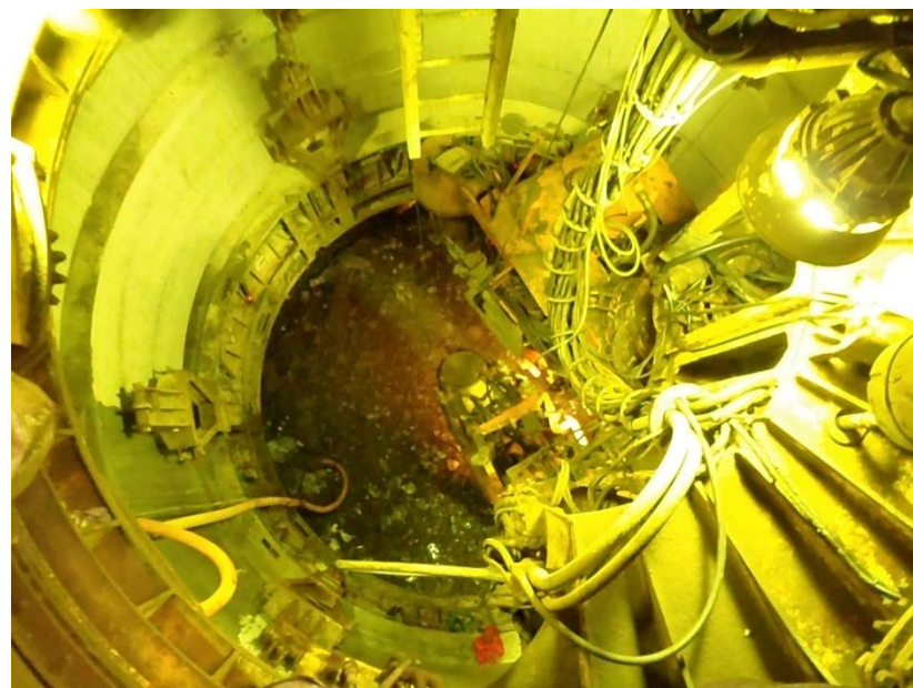
換気立坑の状況 (掘削面を望む)
