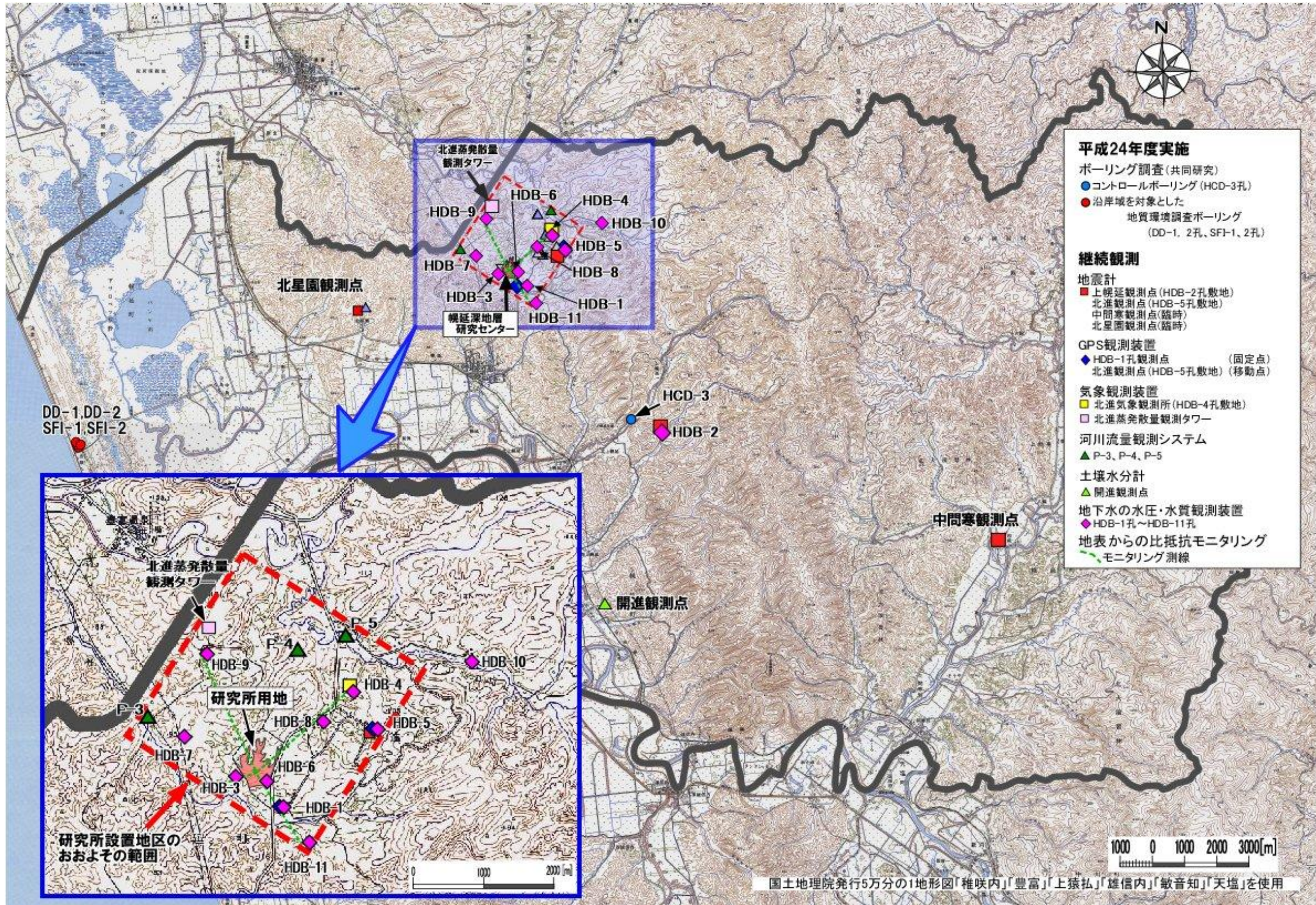
図1 ボーリング孔の位置および観測装置の設置場所
