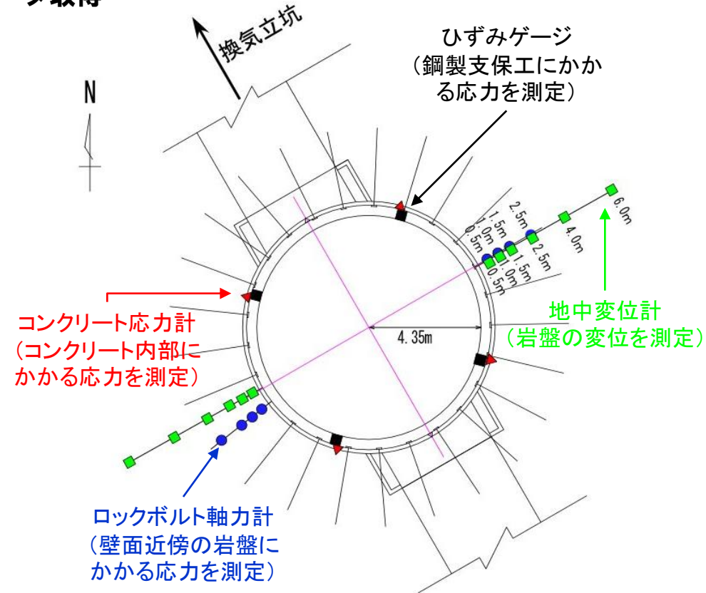
計測機器配置の計画図 (東立坑深度350m)
