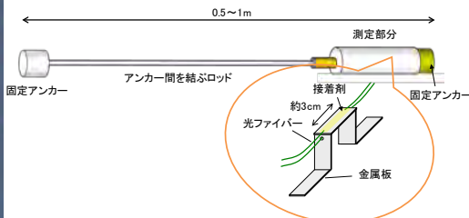
光ファイバー式地中変位計
