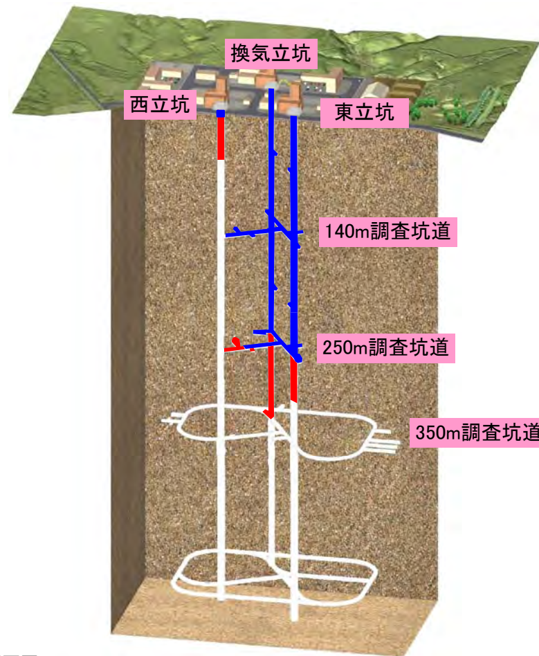
地下施設概要図
