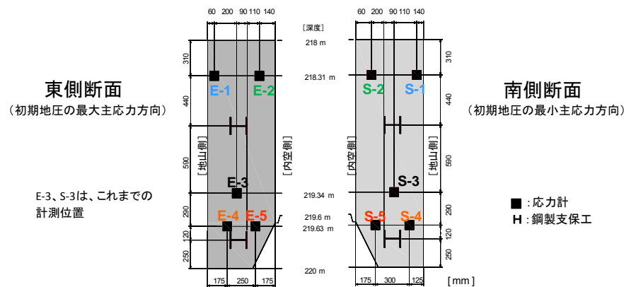
応力計の配置
