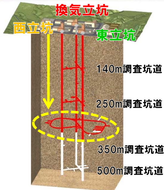
地下施設イメージ図
