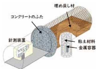
図1 人工バリア性能確認試験のイメージ図
