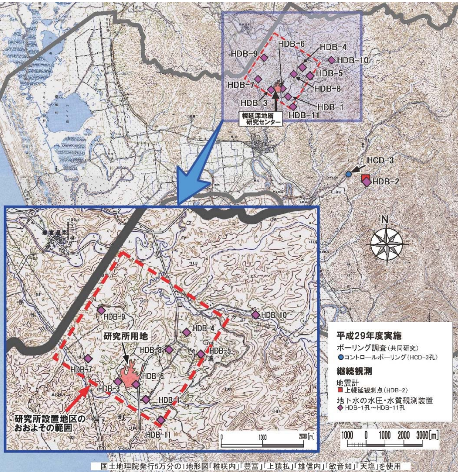
図1 ボーリング孔の位置および観測装置の設置場所
