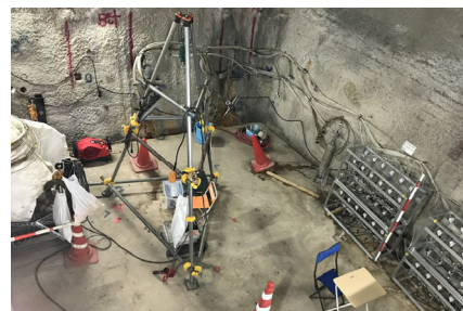
図2 物質移行試験実施状況
