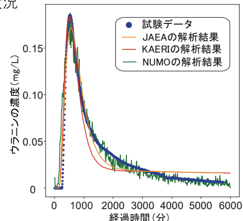
図4 物質移行試験結果と解析での再現結果
