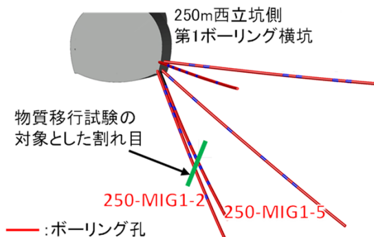
図2 物質移行試験実施状況
