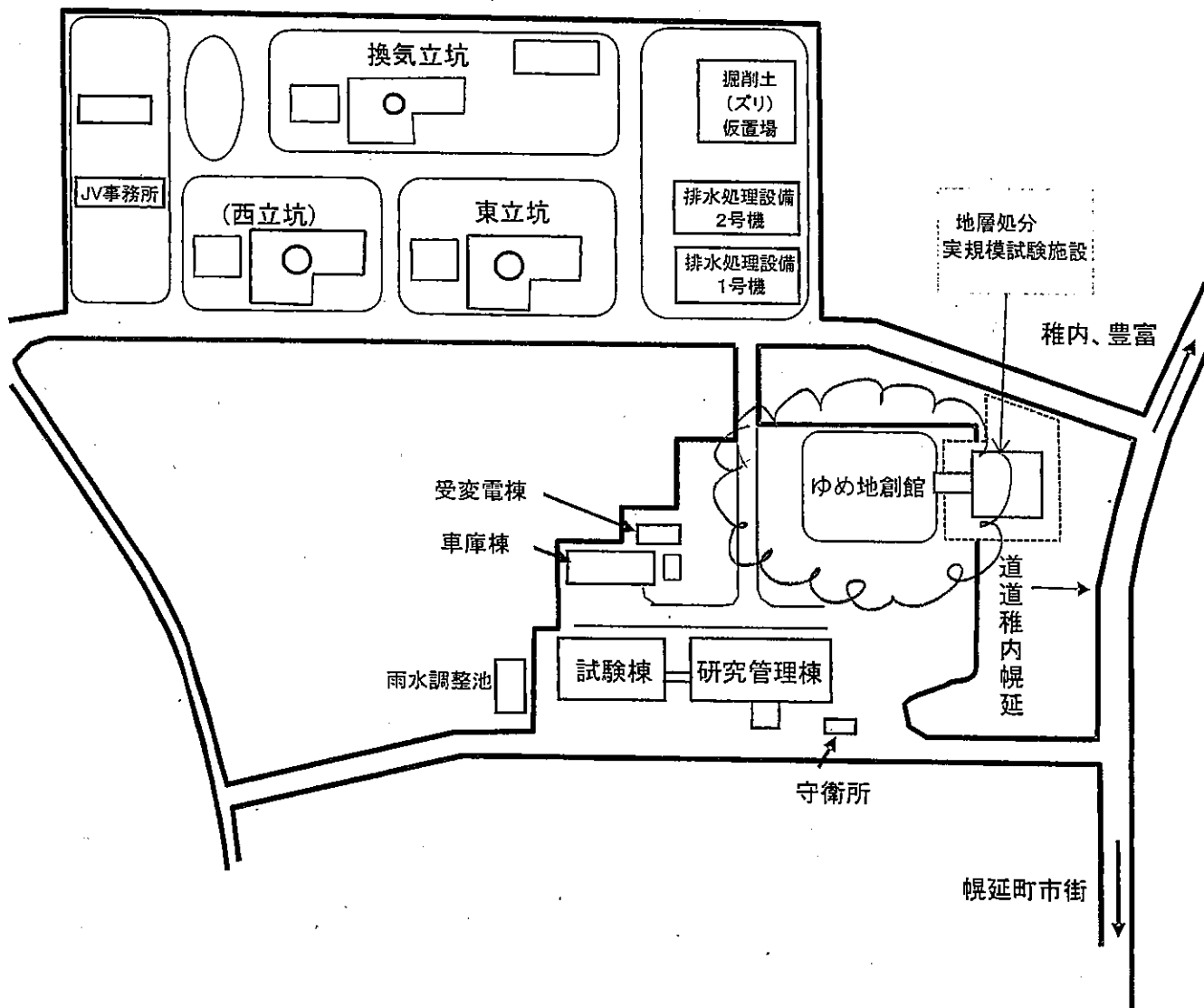
幌延深地層研究センター施設配置図
