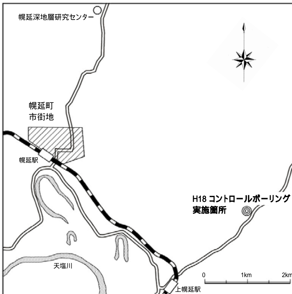
コントロールボーリングの実施箇所
