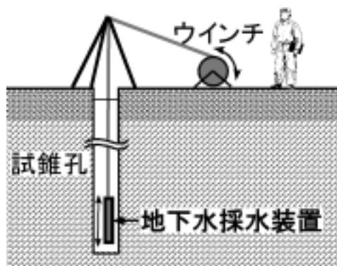
地下水採水作業の例
