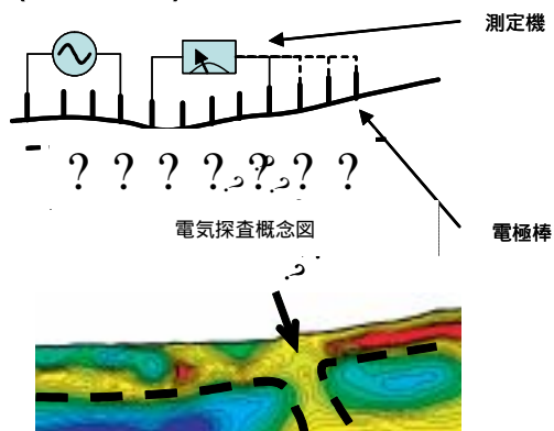
電気探査解析結果の例
