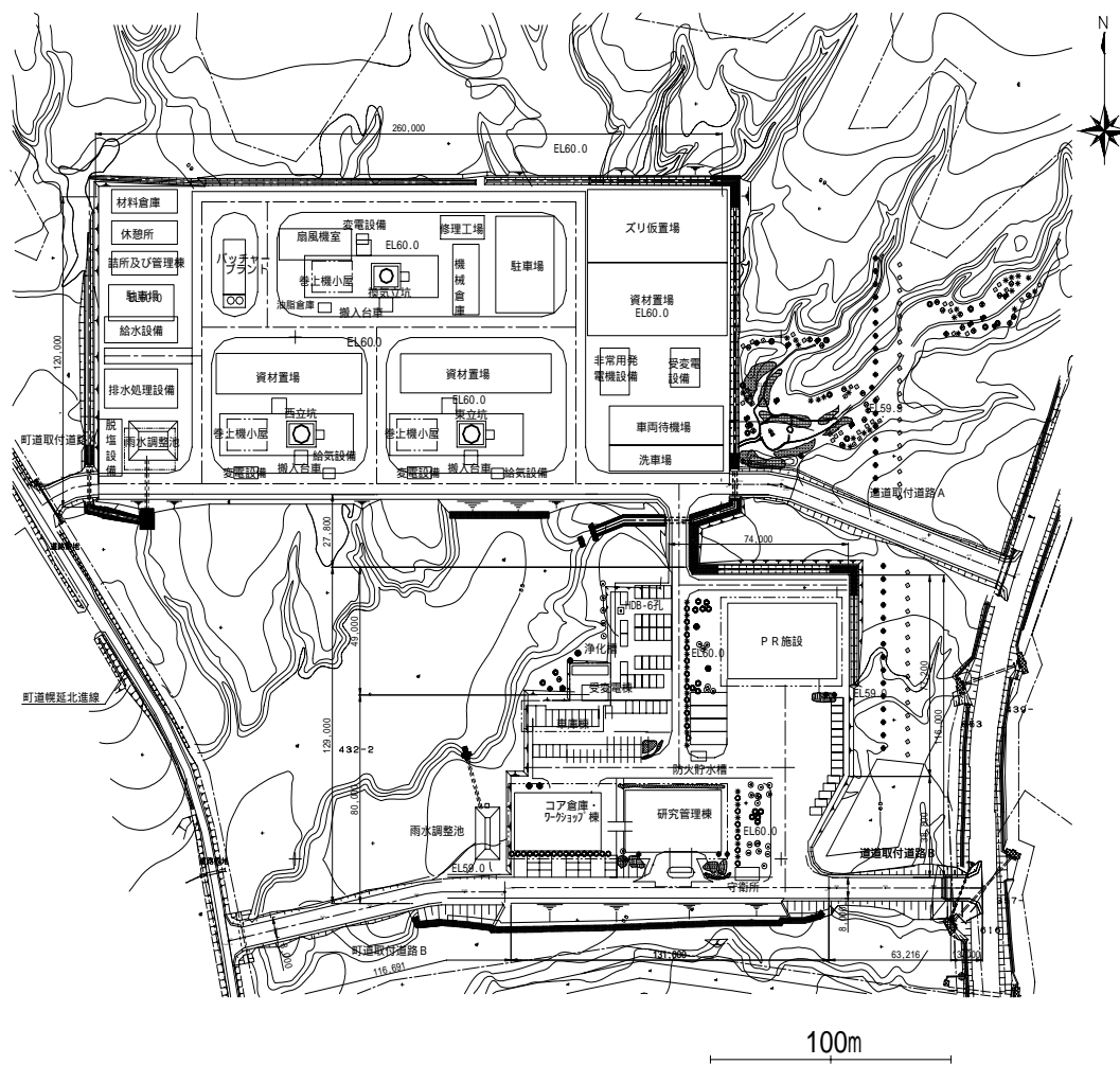
配置計画図
