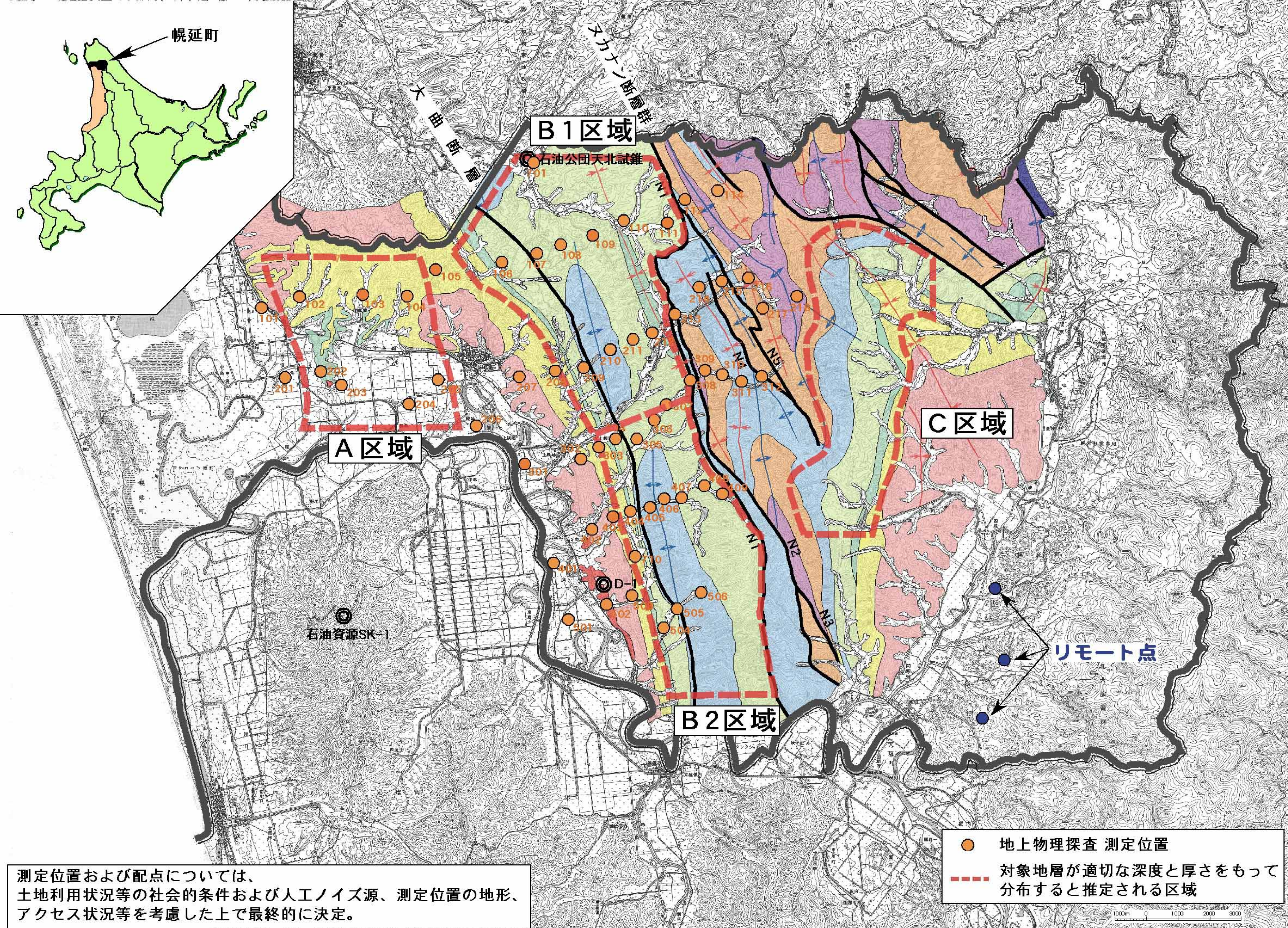
図2 調査範囲図（地上物理探査）
