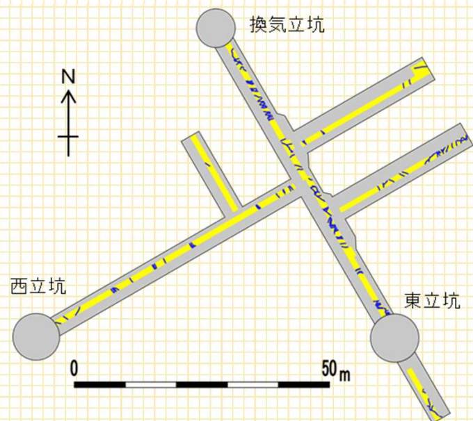
500m調査坑道における断層分布
