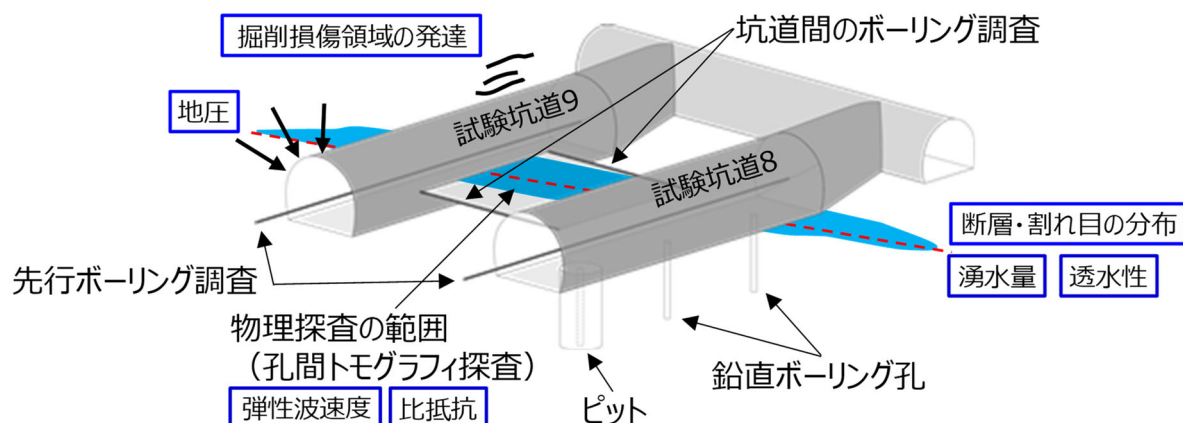
図 21 500m 調査坑道の試験坑道 8 および試験坑道 9 における原位置調査のイメージ図
