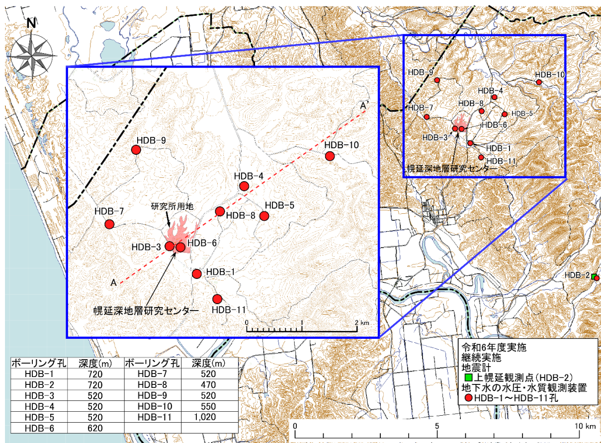
図 4 ボーリング孔の位置および観測装置の設置場所
