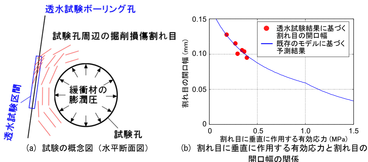
図 24 試験孔周辺に発達した掘削損傷割れ目を対象とした透水試験の概念図と割れ目に作用する有効応力と開口幅の関係 (9)
