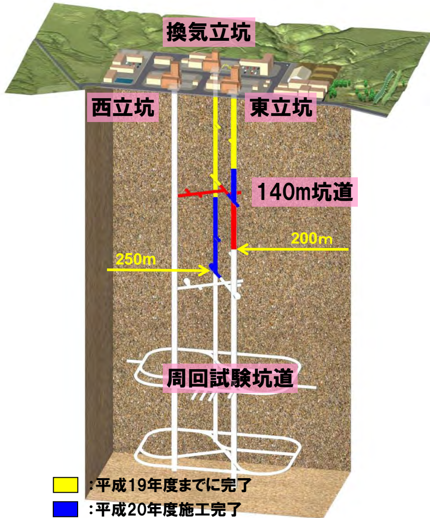
地下施設配置図
