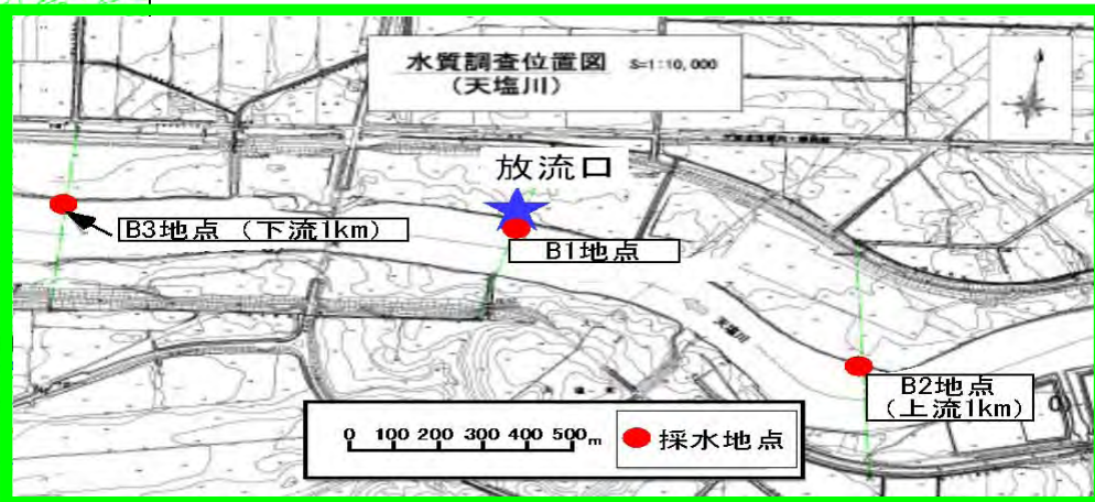
天塩川放流口詳細位置図
