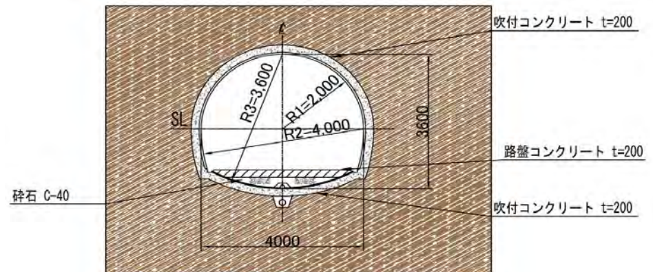
水平坑道
