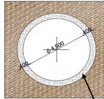
換気立坑
