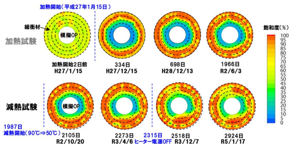
飽和度の時間変化（比抵抗トモグラフィ）
