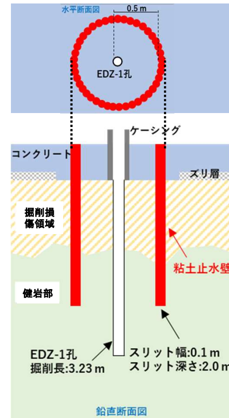
試験概念図
