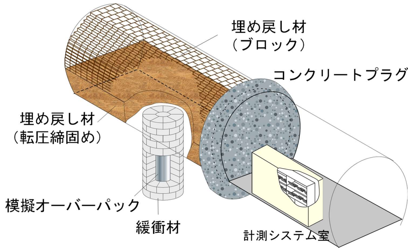
人工バリア性能確認試験（試験坑道4）の概念図
