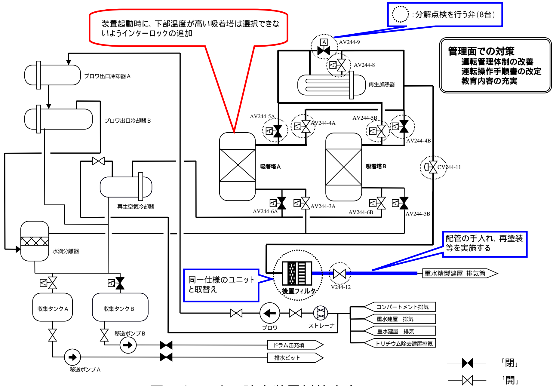
図-3 トリチウム除去装置対策内容
