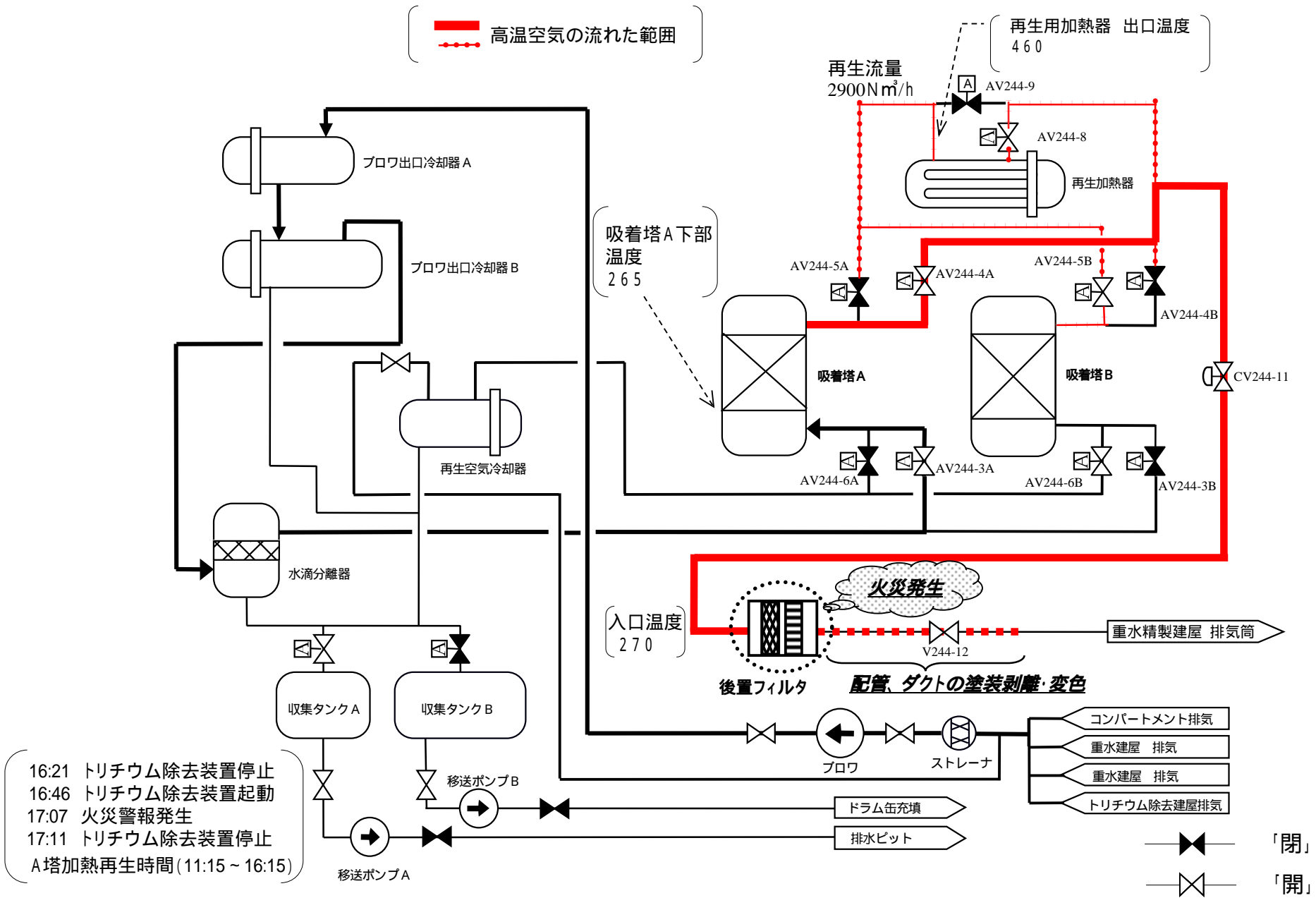
図-1 トリチウム除去装置火災発生時の状況
