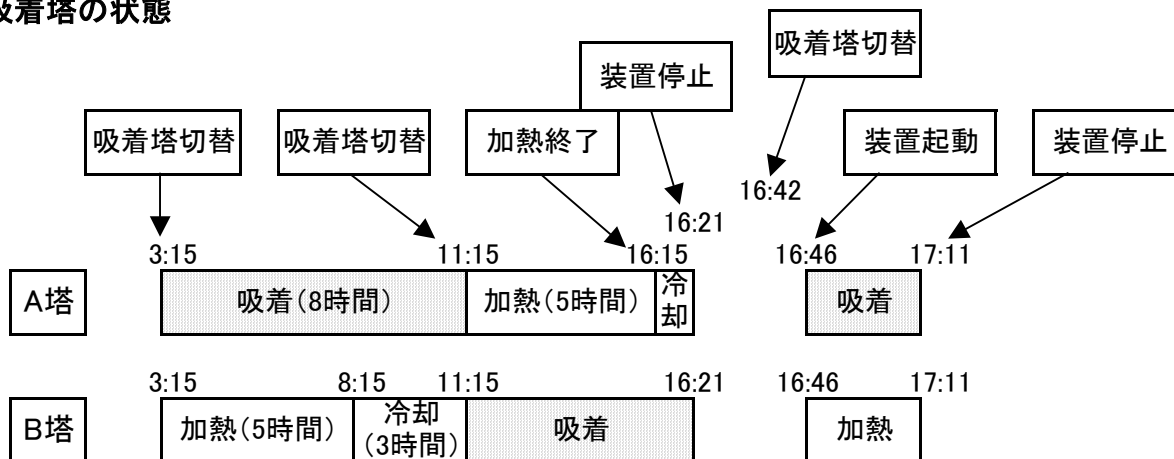
図-6 トリチウム除去装置の運転サイクル
