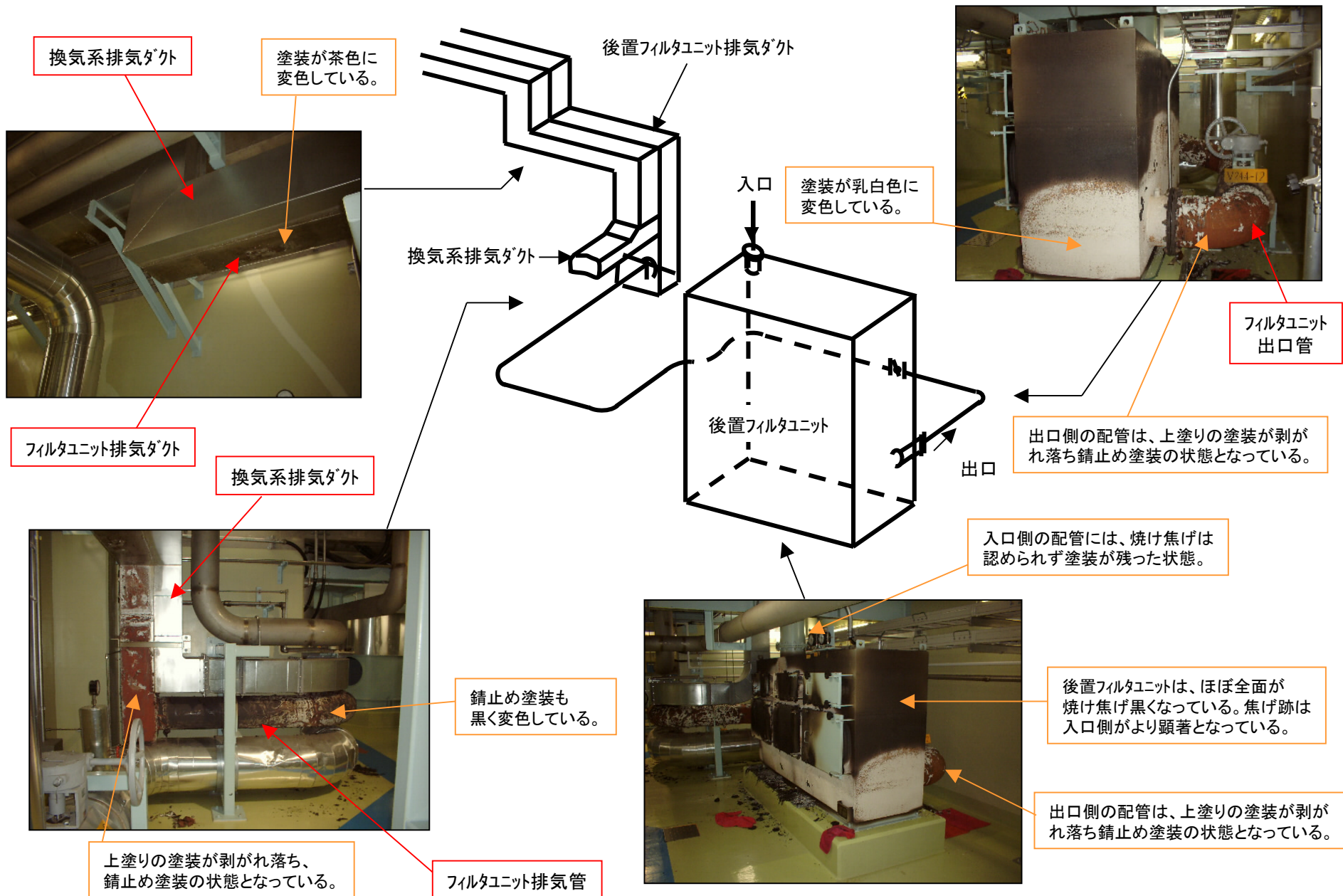
図-4 後置フィルタユニット焼損状況
