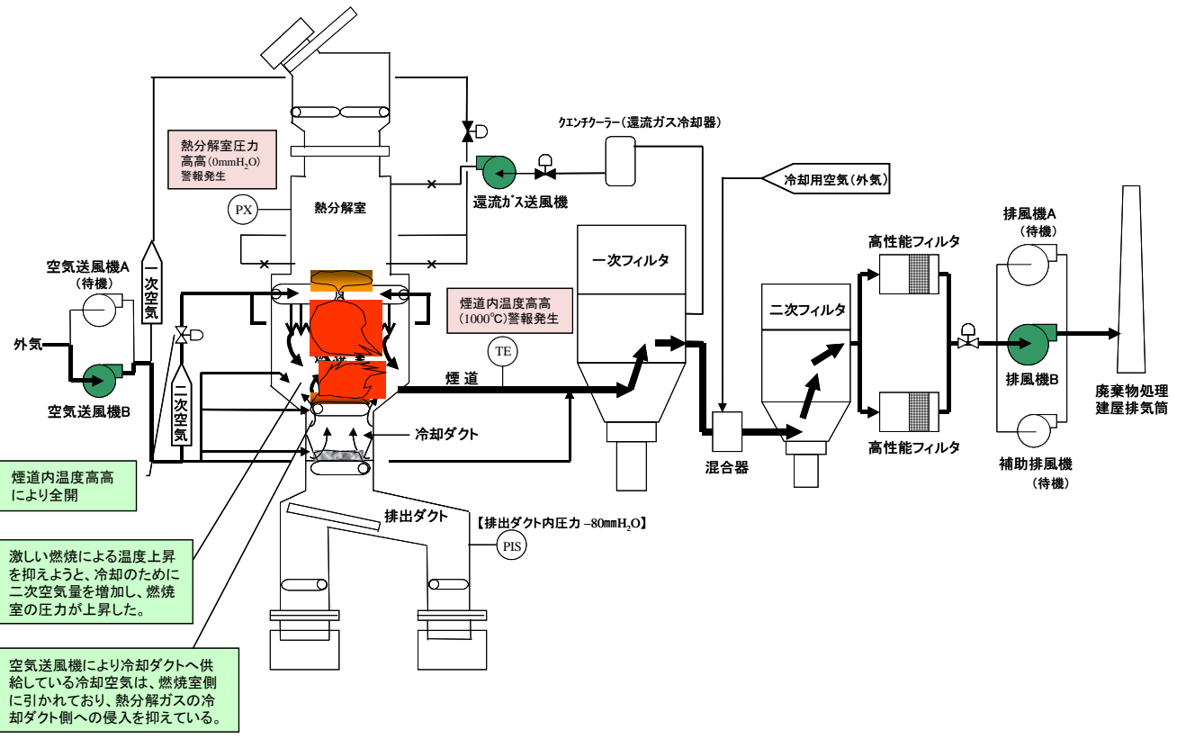
② 熱分解室圧力高高(0mmH 2 O)、煙道内温度高高(1000℃)警報発生時
