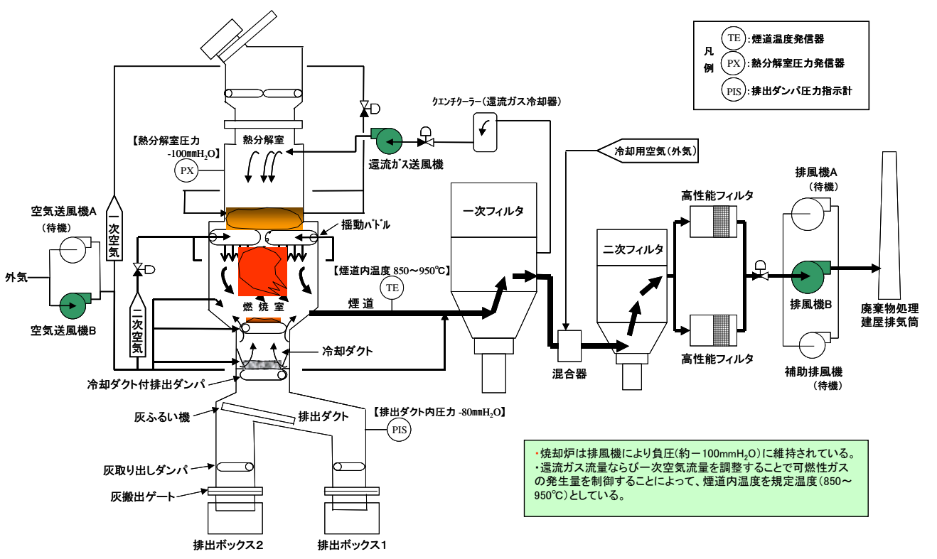
① 通常の運転状態
