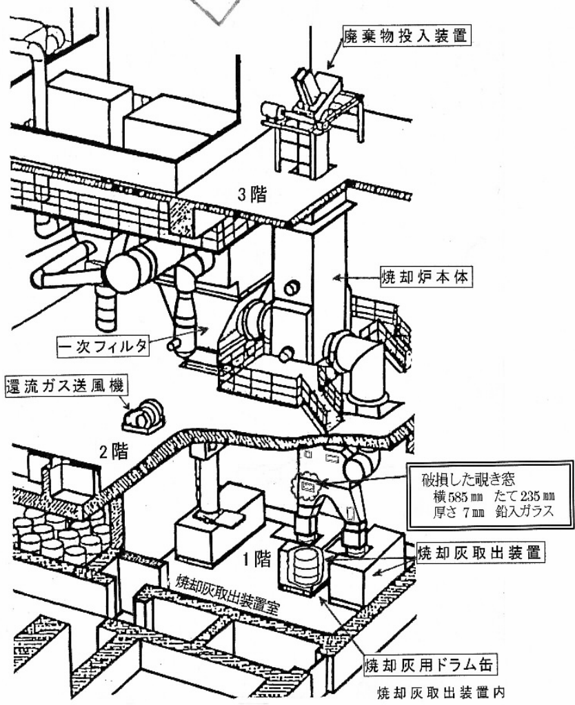
廃棄物処理建屋鳥瞰図 (拡大)
