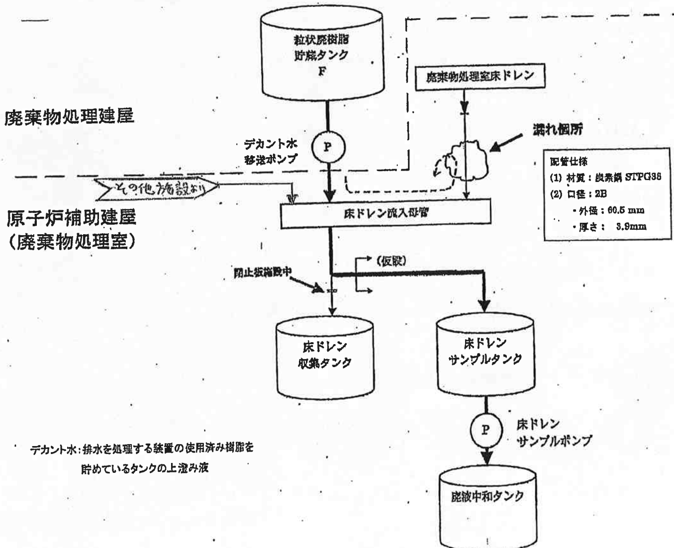
全体機器配置図 (廃棄物処理室 地下1階)
