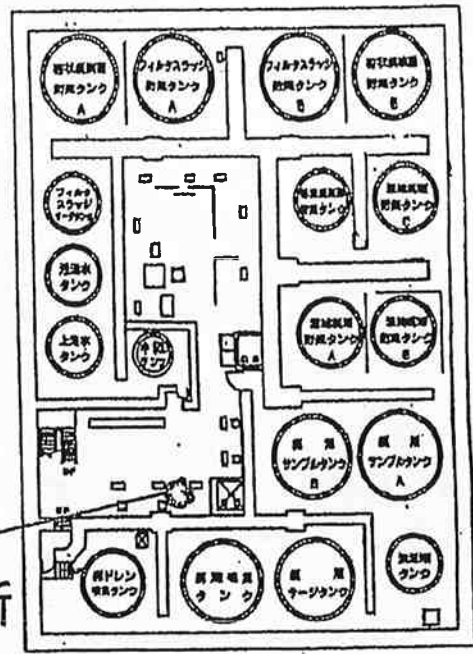
廃棄物処理室平面図(地下1階)
