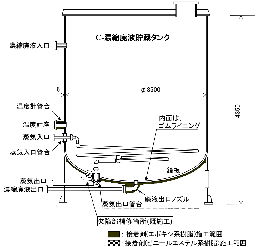
タンク底部(鏡板全面)エポキシ系樹脂施工図
