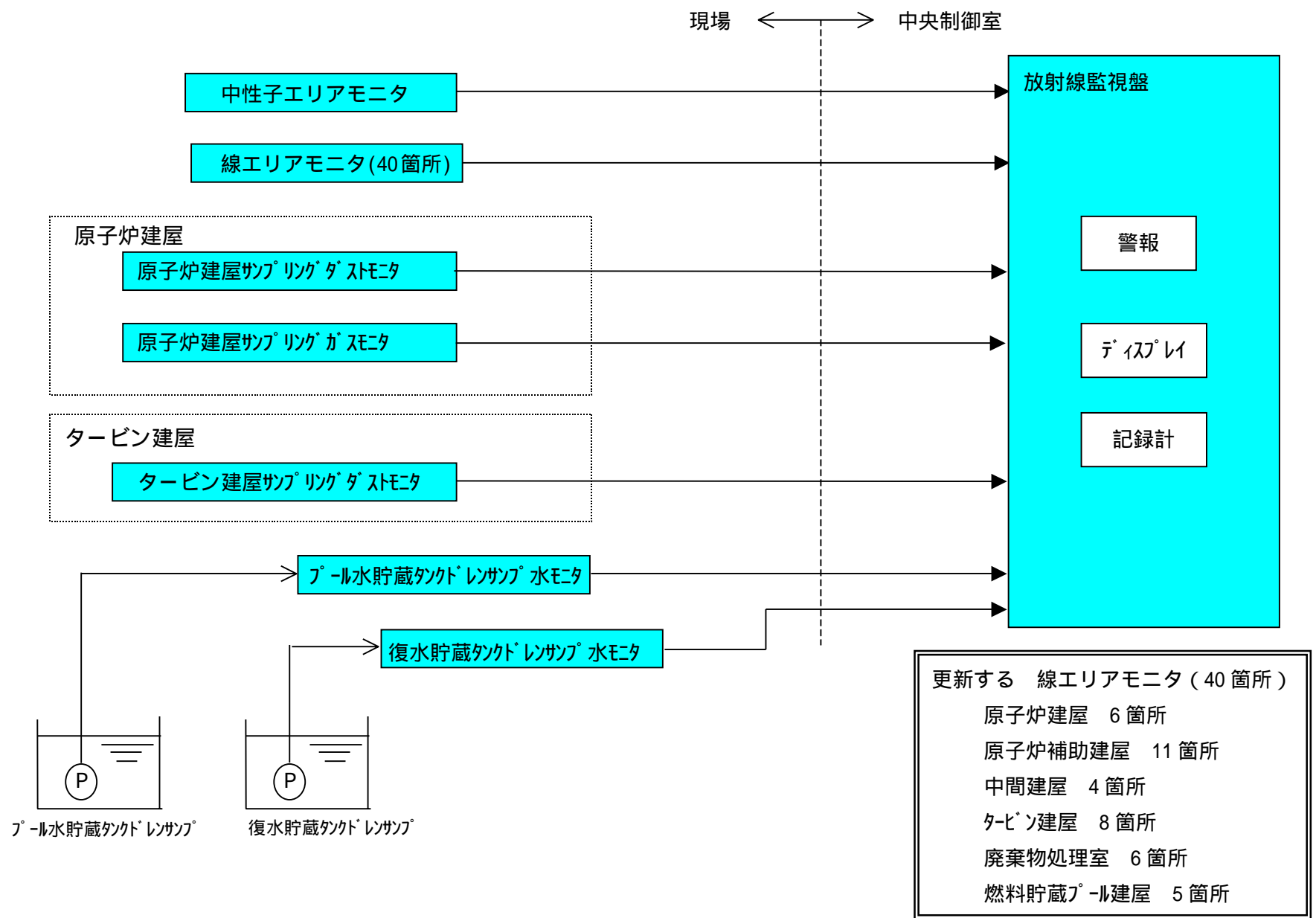
図-2 プロセス放射線監視装置の変更工事概要
