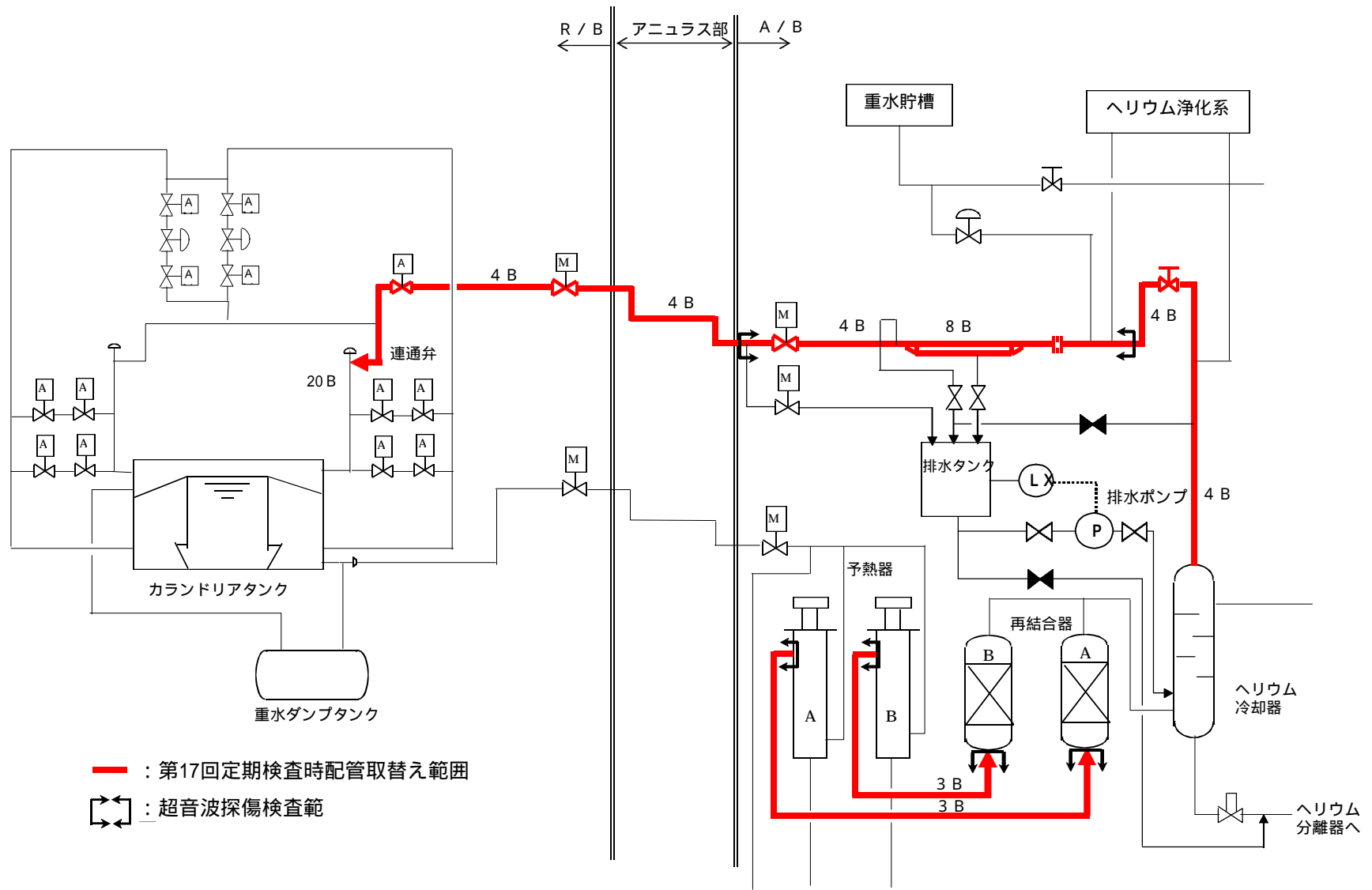
図-2 ヘリウム循環系配管超音波探傷検査箇所
