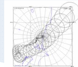
流跡線ガウスパフモデルの概念図
