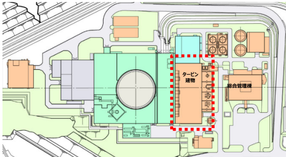
もんじゅ建物配置
