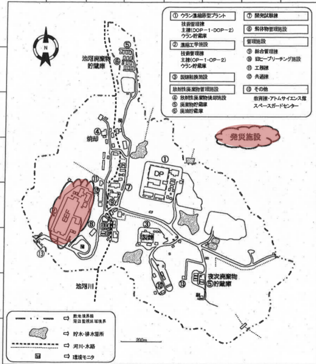
人形峠環境技術センター 敷地配置図
