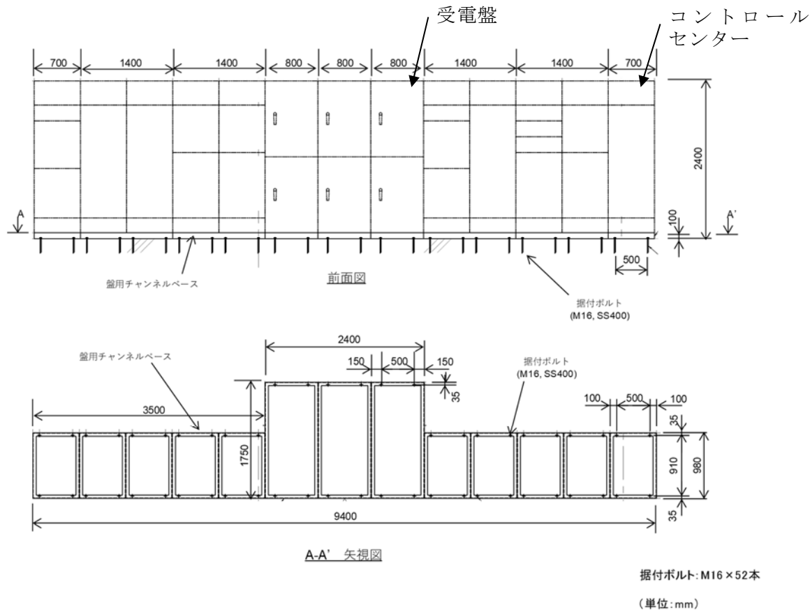
電源接続盤構造図
