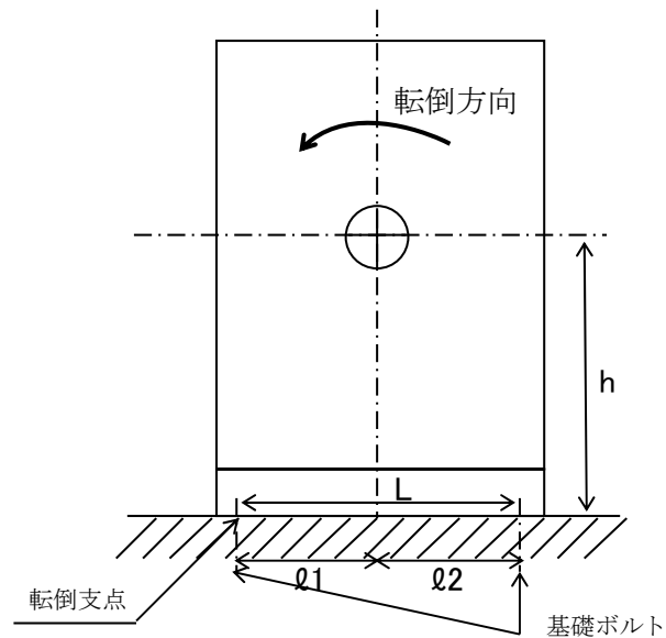
計算モデル
