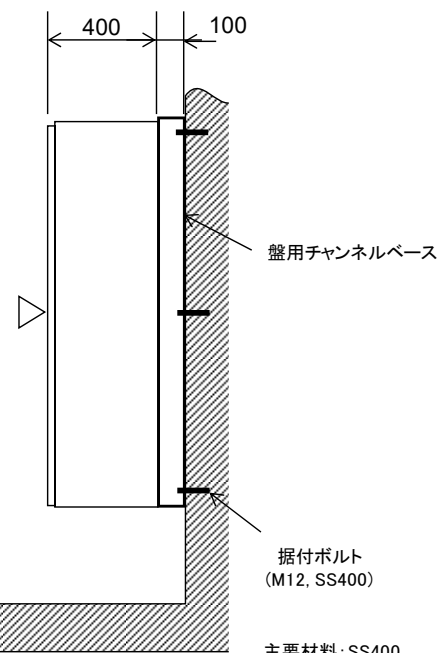
側面図
