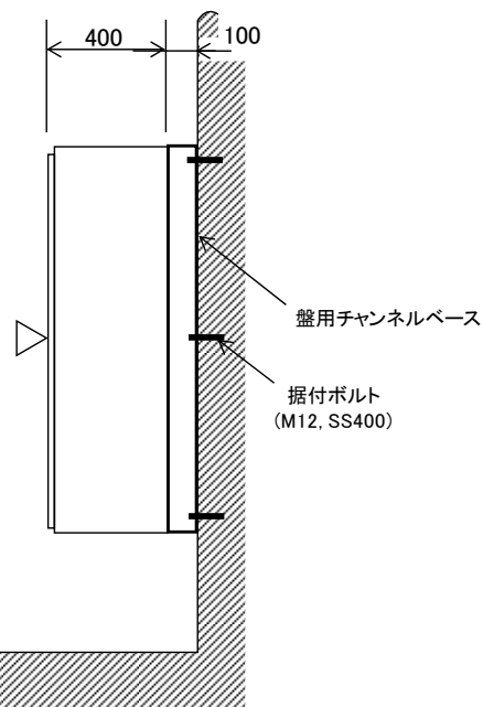
側面図
