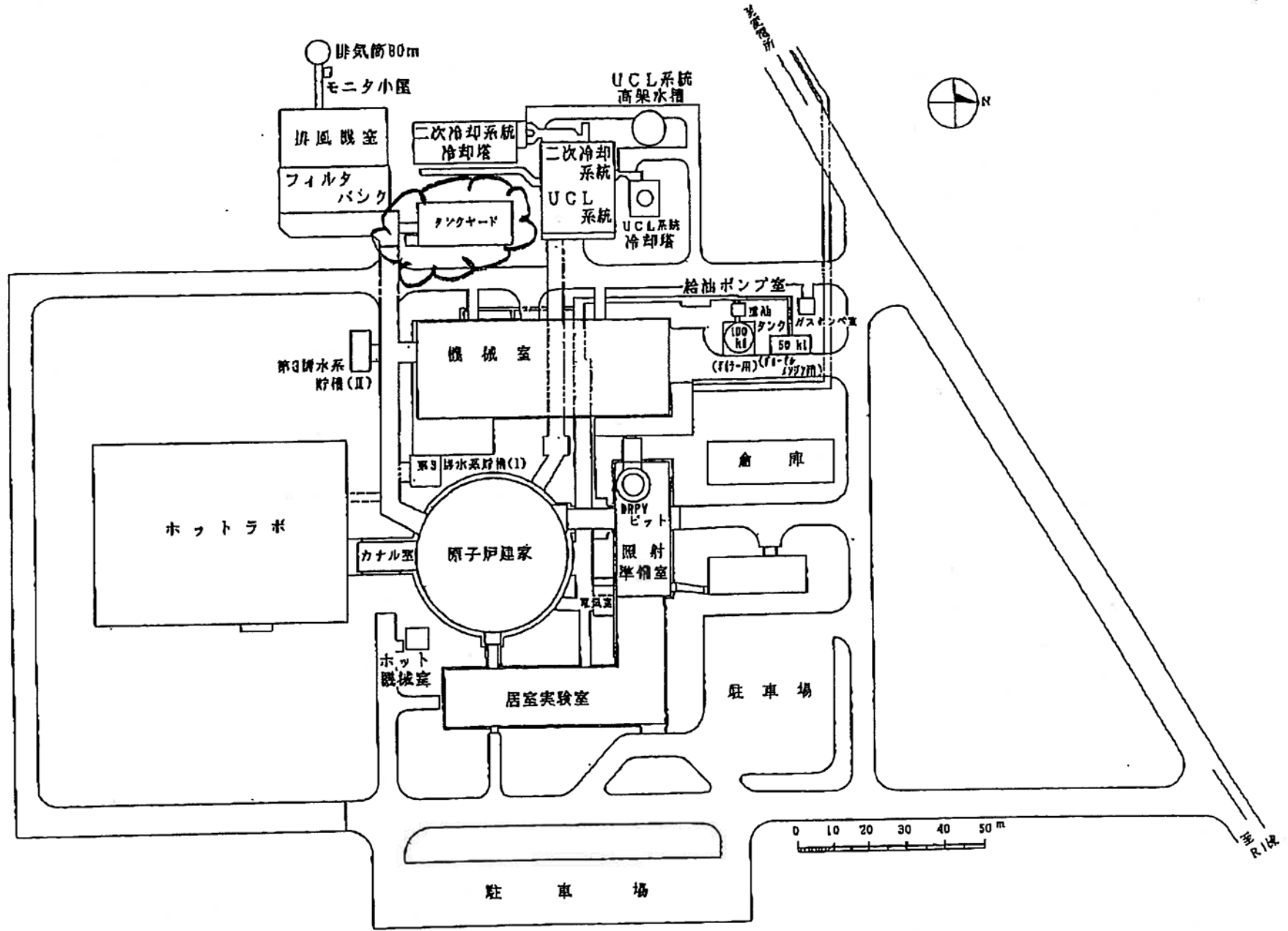
第1図 JMTR建家配置図
