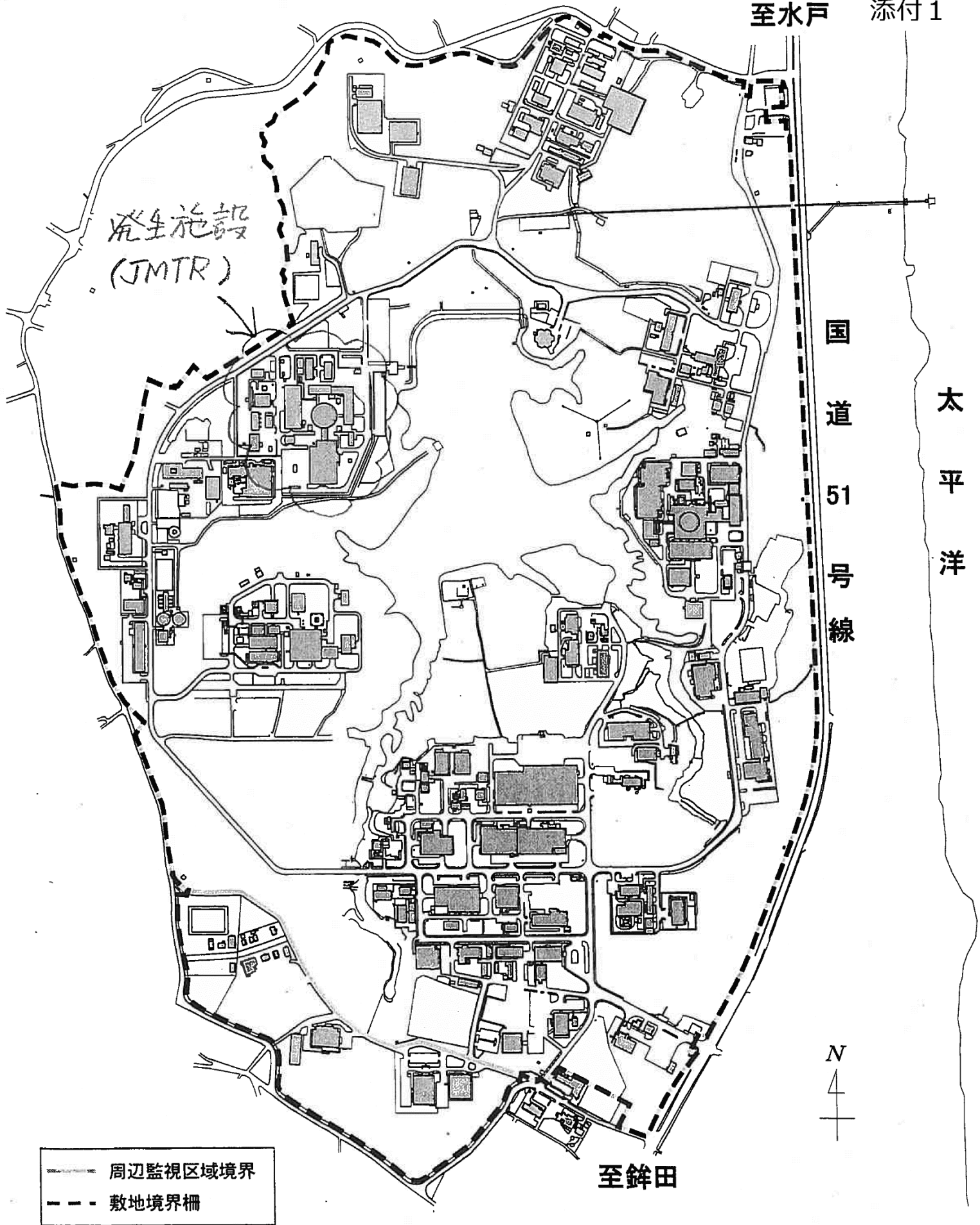
大洗研究所 施設配置図
