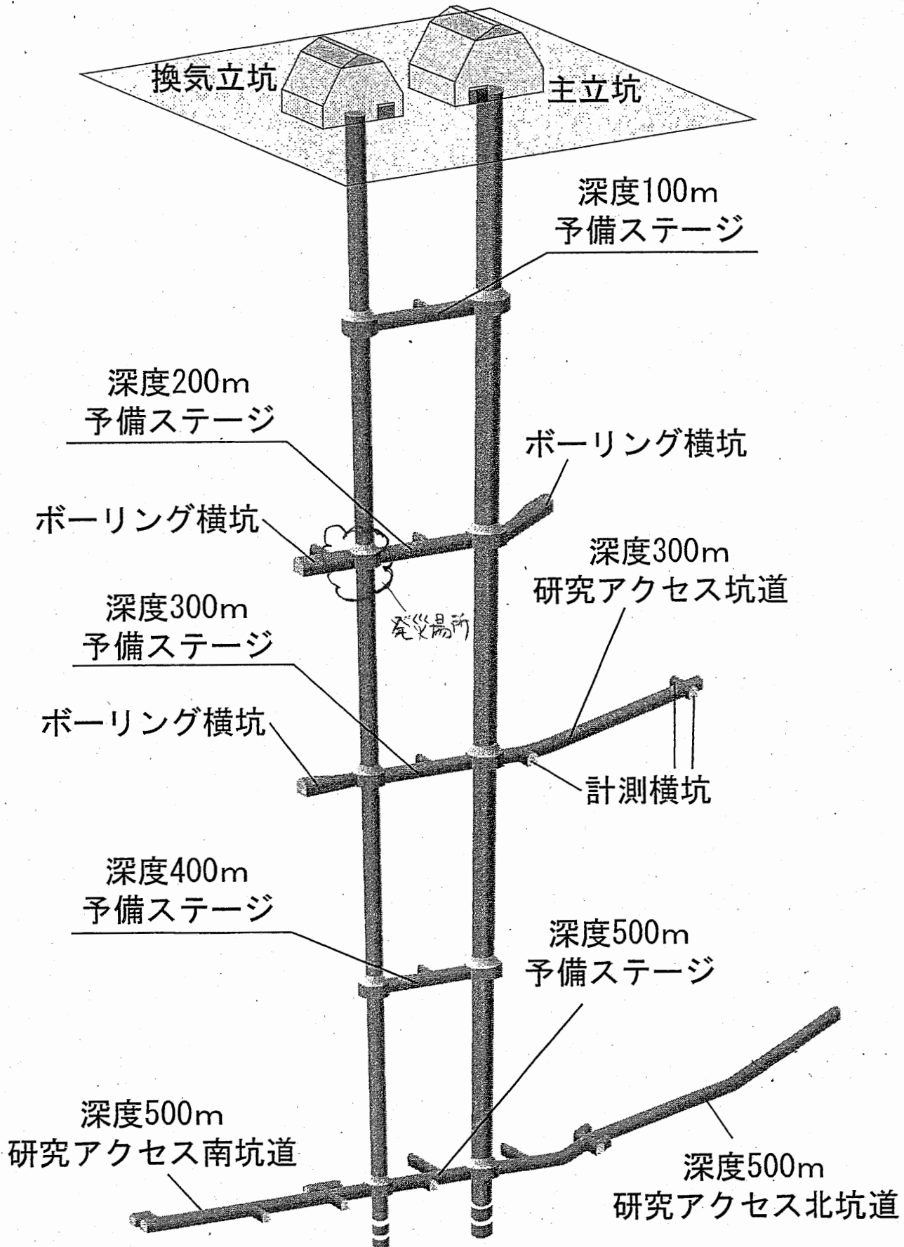
研究坑道イメージ図
