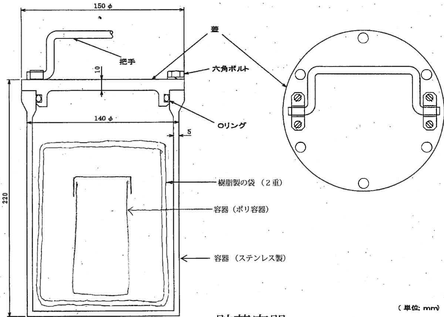
貯蔵容器
