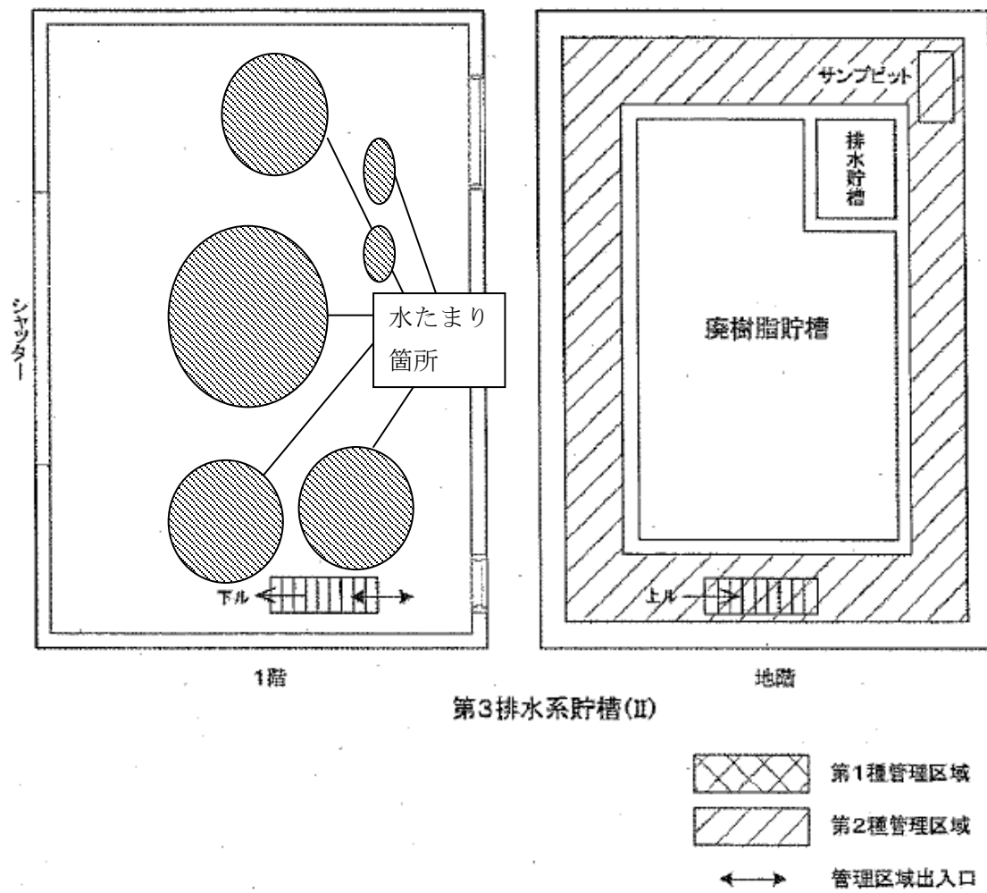
図3 第3排水系貯槽(Ⅱ) 平面図
