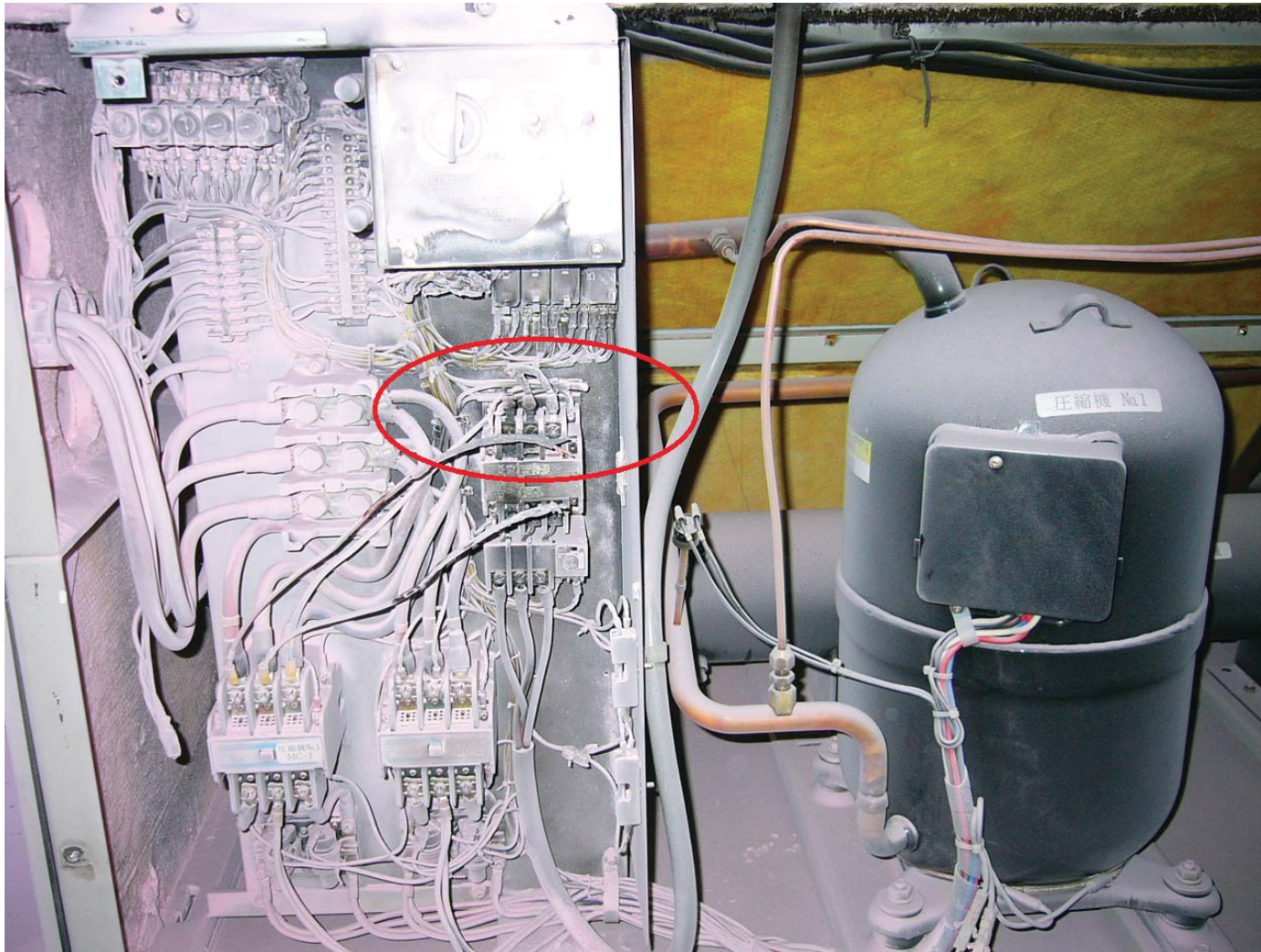
図3 パッケージエアコンの焼損箇所
