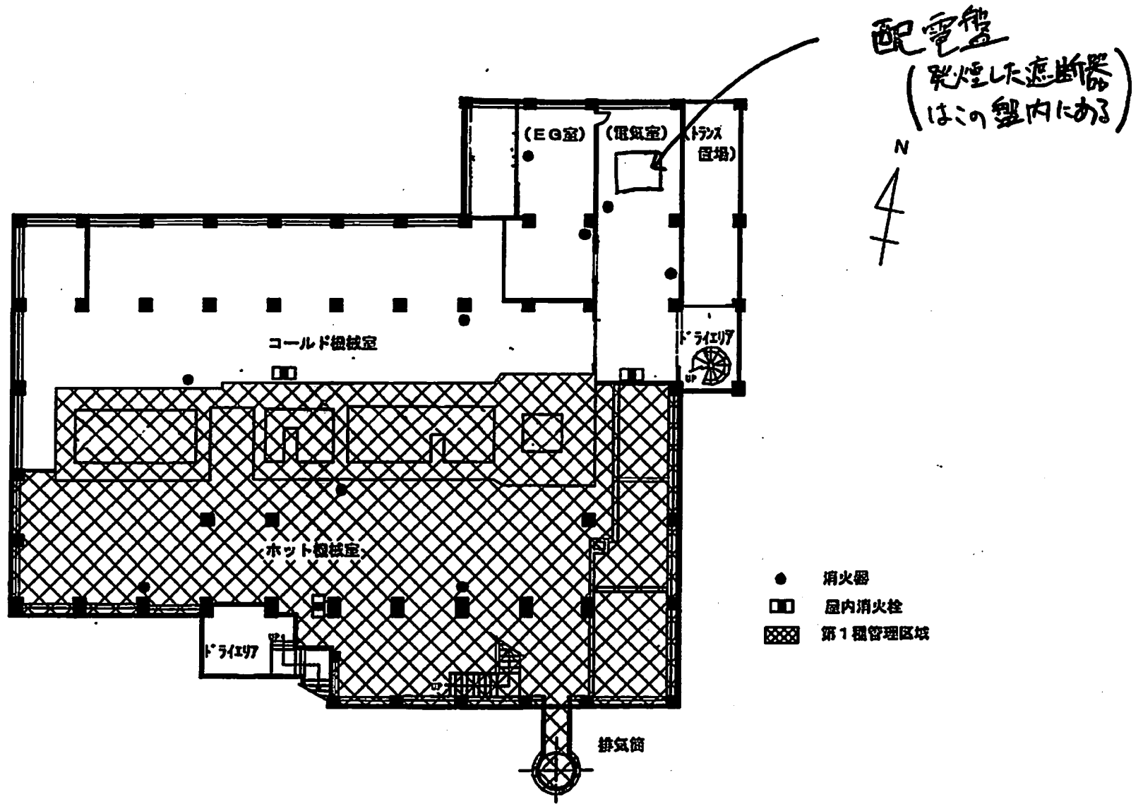
廃棄物安全試験施設の消火設備配置図 (地階)
