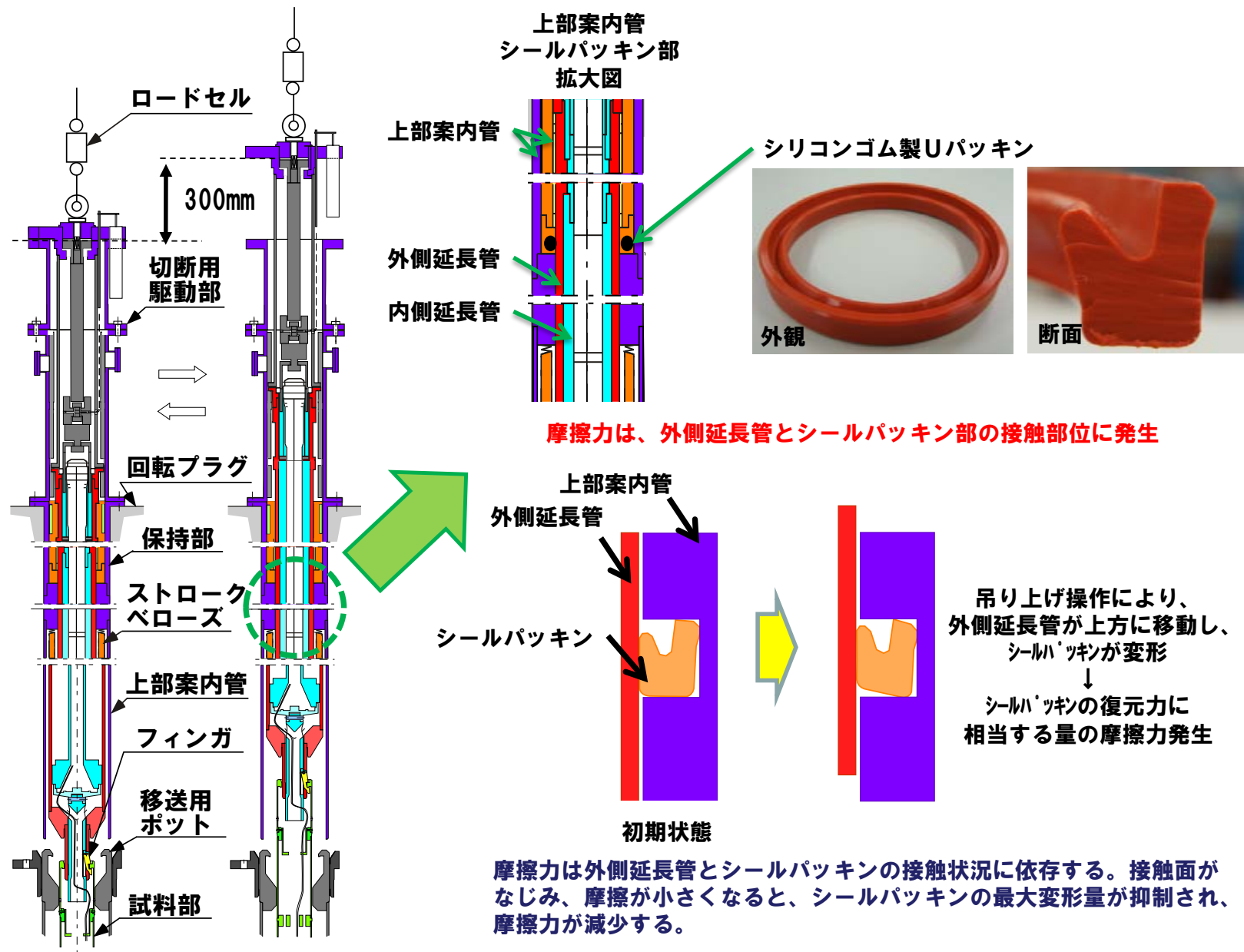
図-5 MARICO-2 における摩擦力発生部位
