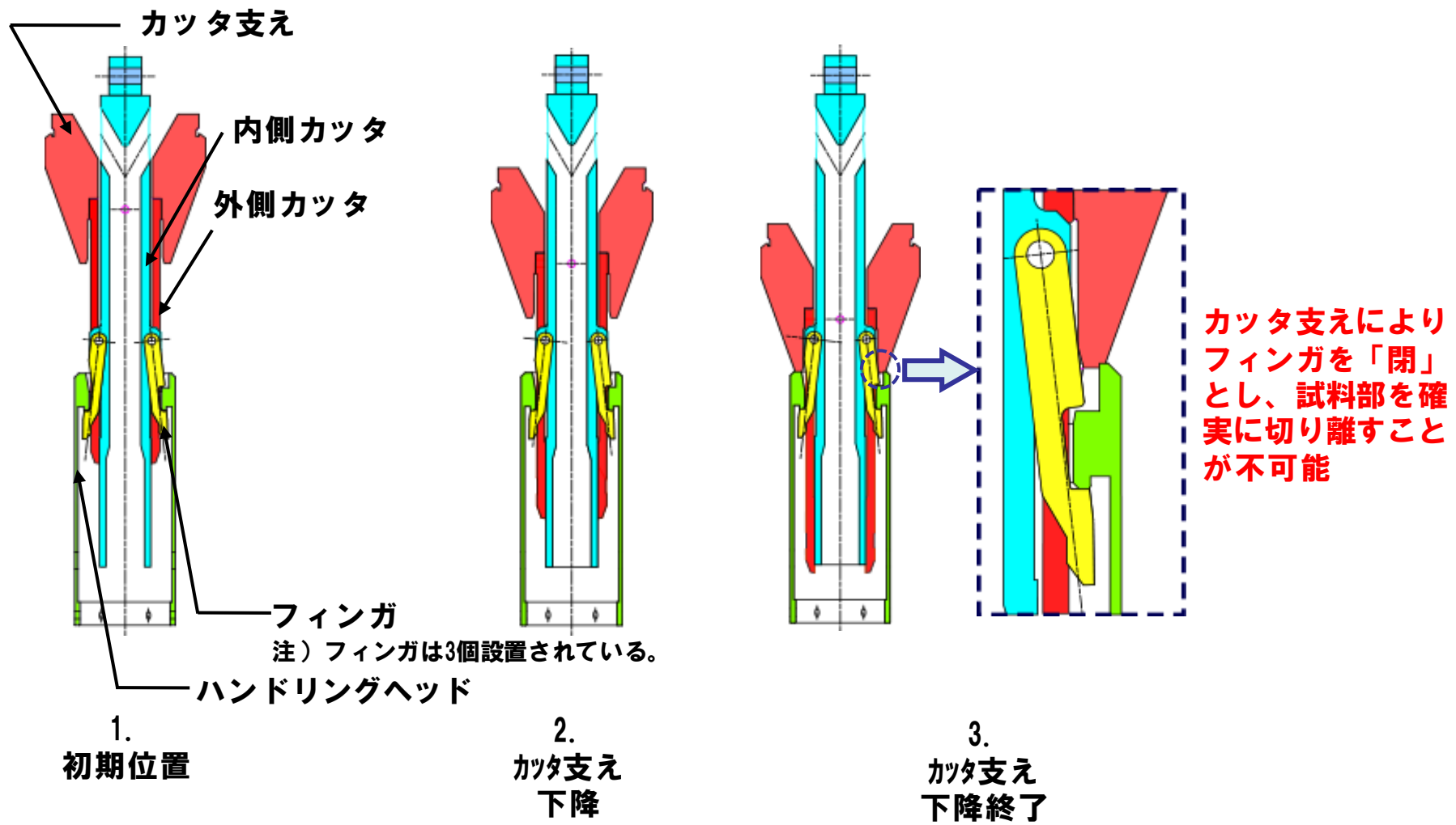
図-4 MARICO-2 試料部切離機構設計精査結果
