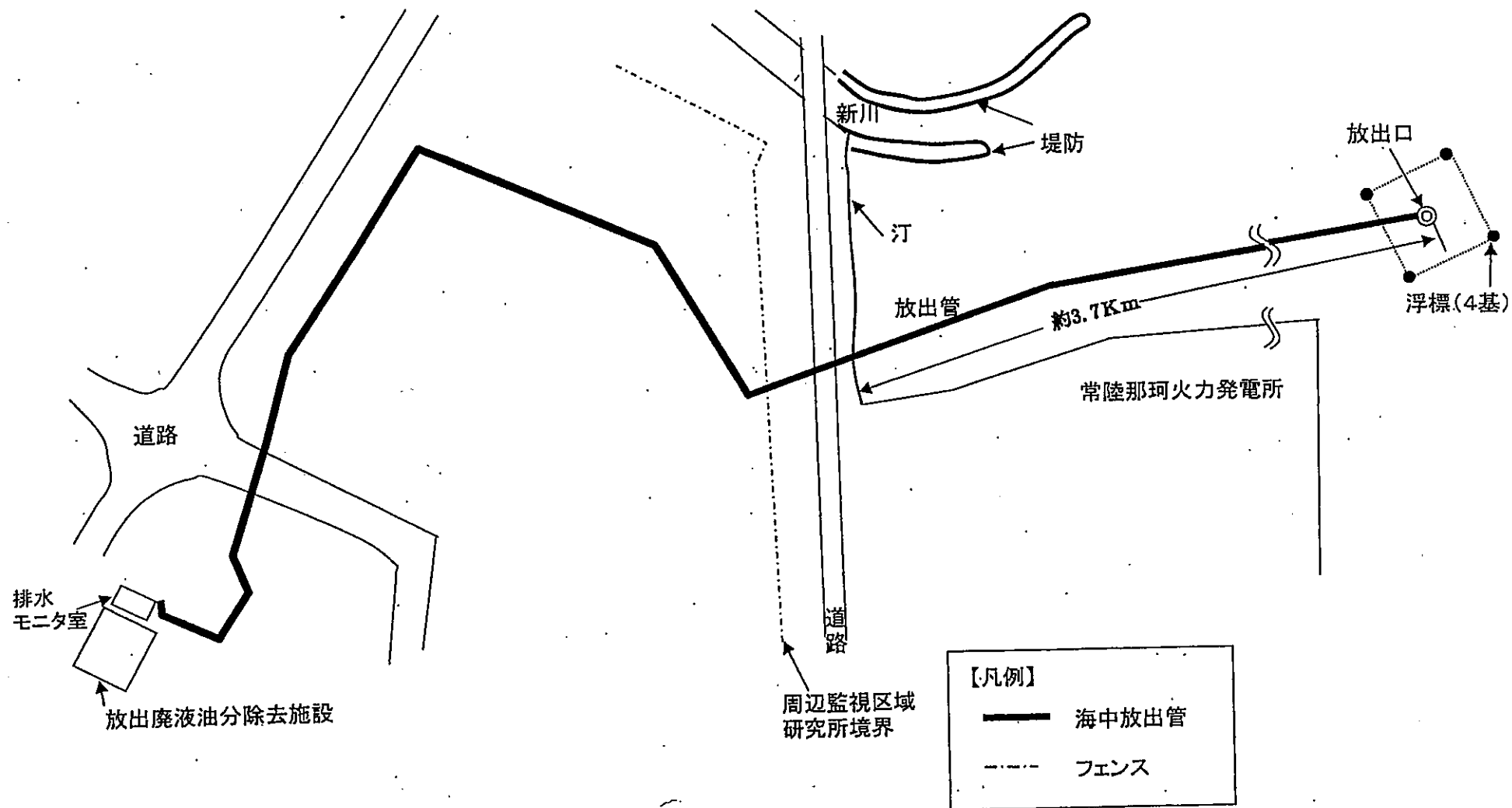
海中放出管経路概略図
