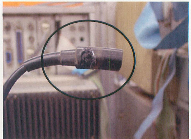
電源供給用プラグ
