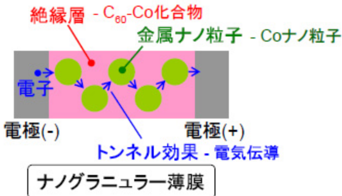
図4 ナノグラニューラー薄膜のTMR効果 模式図
