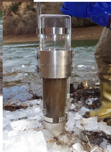
柱状堆積物試料の採取 (不攪乱柱状採泥器)
