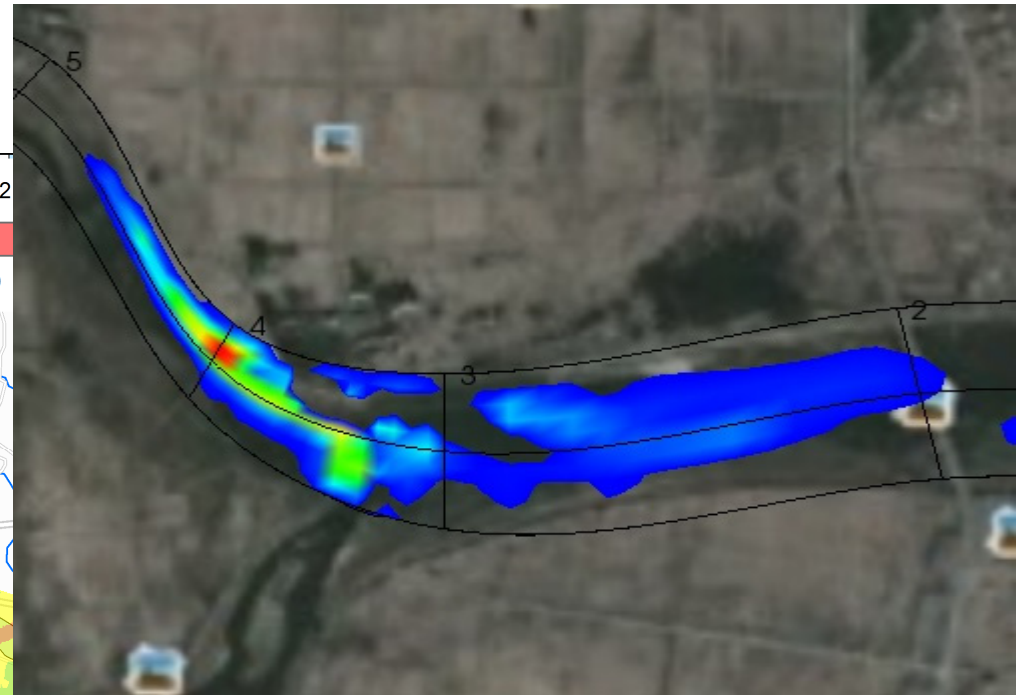
輸送土砂の集積
