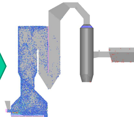
焼却灰のセシウム挙動解析
