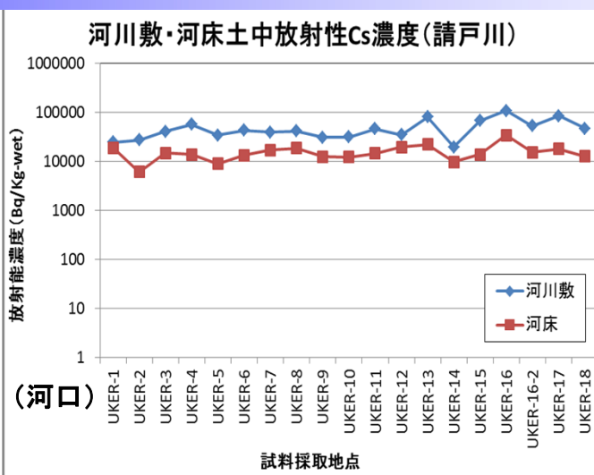
小高川(左図)及び請戸川(右図)の河川敷・河床土中の放射性セシウム濃度
