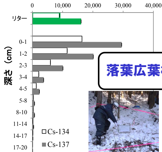
放射性セシウム濃度 (Bq/kg)
