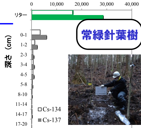
放射性セシウム濃度 (Bq/kg)
