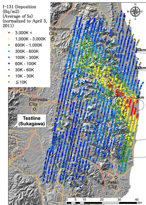
実測値に基づくヨウ素131の分布
