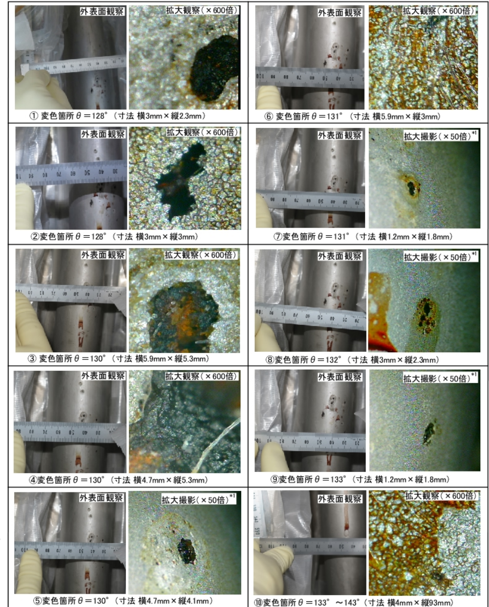
図-2 ベローズ概要と外表面観察結果
