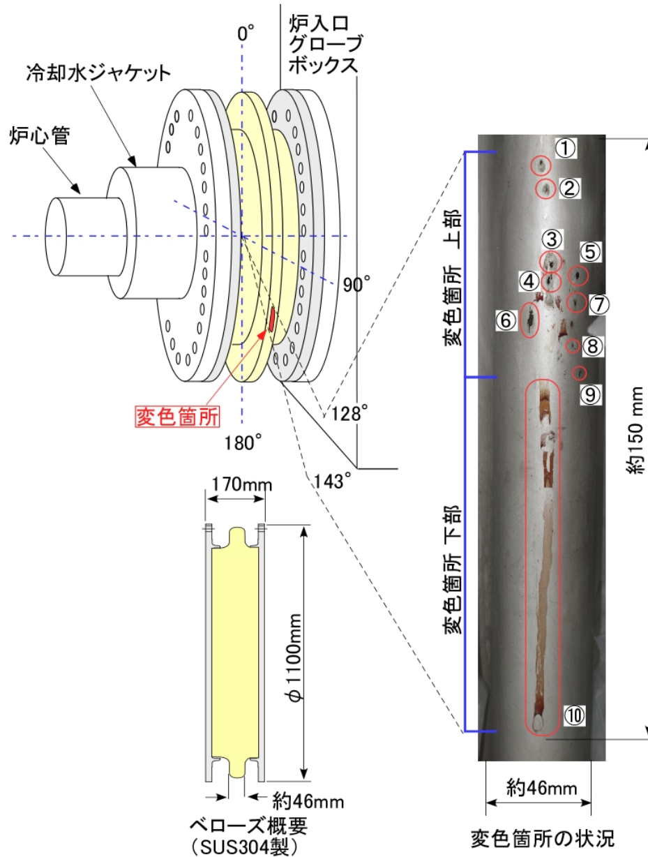
図-2 ベローズ概要と外表面観察結果
