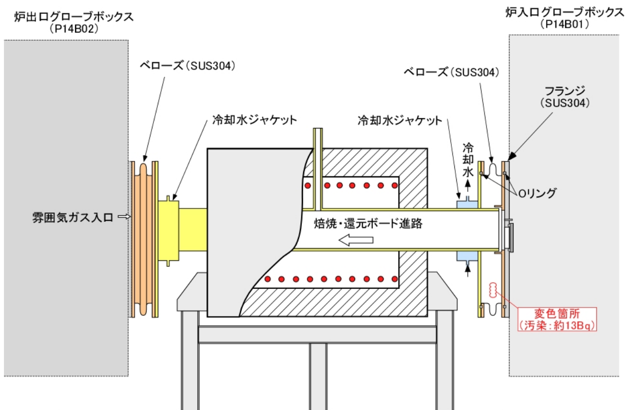
焙焼還元炉の概要図
