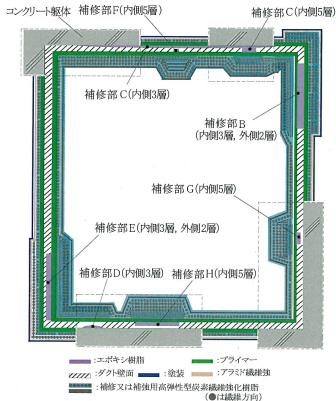
図-2 主排気筒ダクト補修箇所断面図
