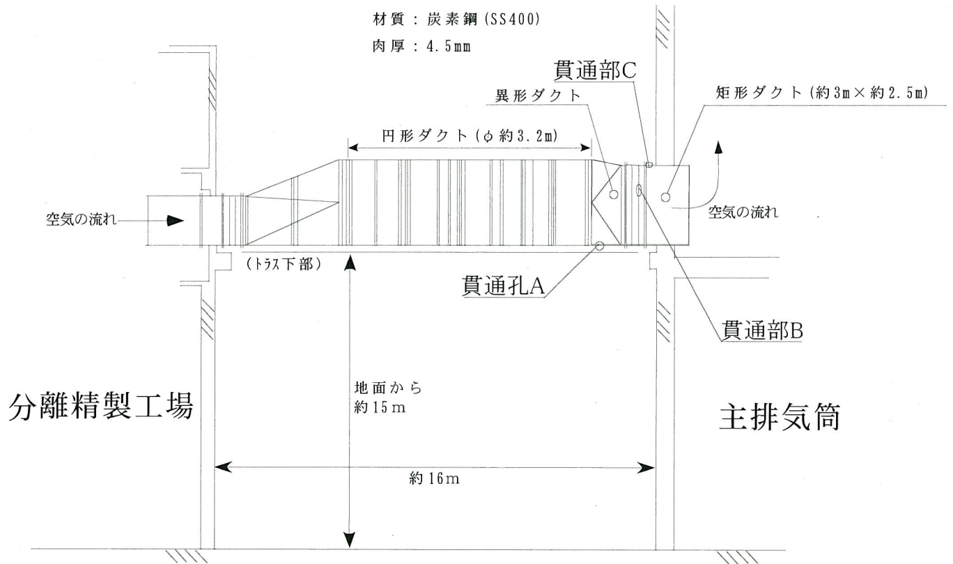
図-1 主排気筒ダクト貫通孔概要図
